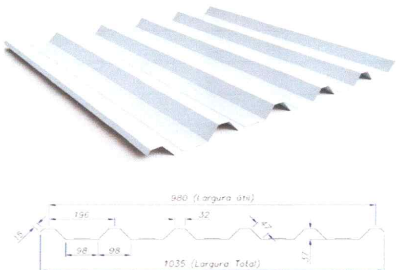
Figura 11 – imagem telha metálica trapezoidal TP40-980
