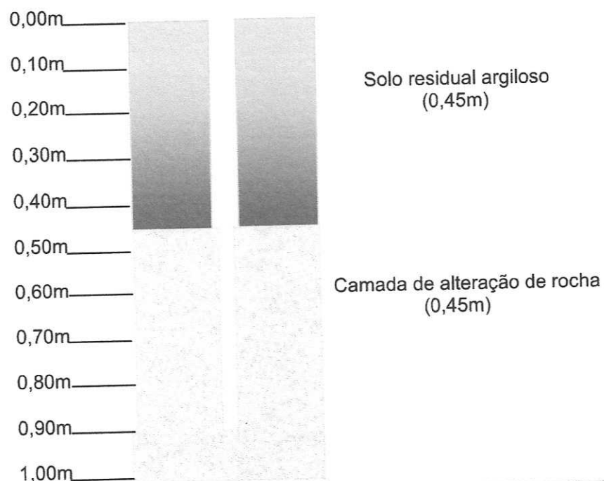
Fig. 02: Perfil esquemático em SP 02 com profundidade final de 0,90.
