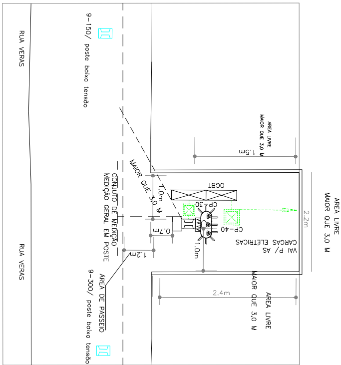
PLANTA BAIXA – SUBESTAÇÃO ESCALA: 1/75
