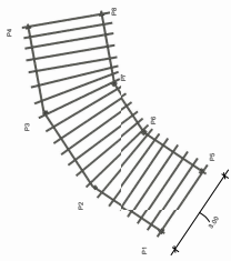
② DETALHAMENTO CARAMANCHÃO 1: 100
