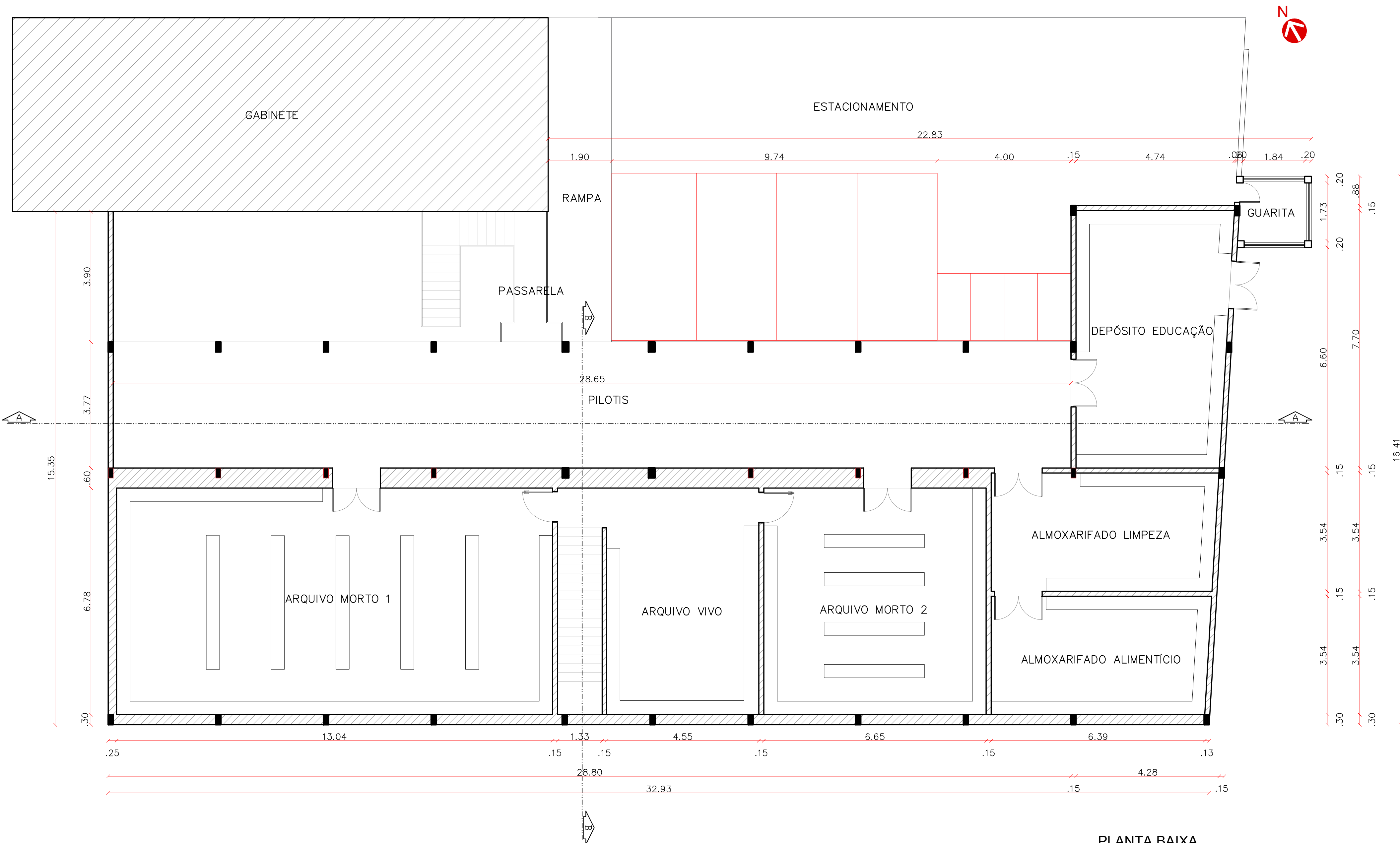
PLANTA BAIXA LAYOUT SUBSOLO
