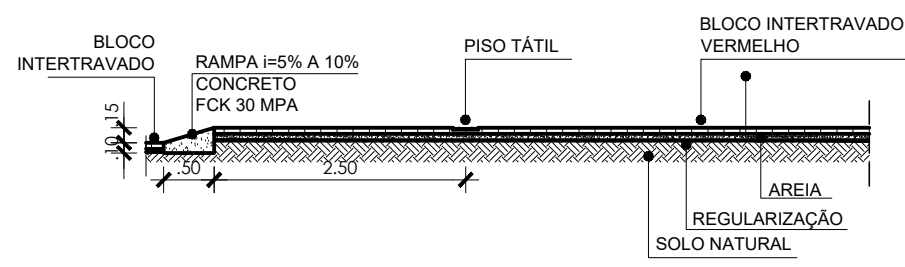
2 CORTE AA- FAIXA ELEVADA ESCALA 1:75
