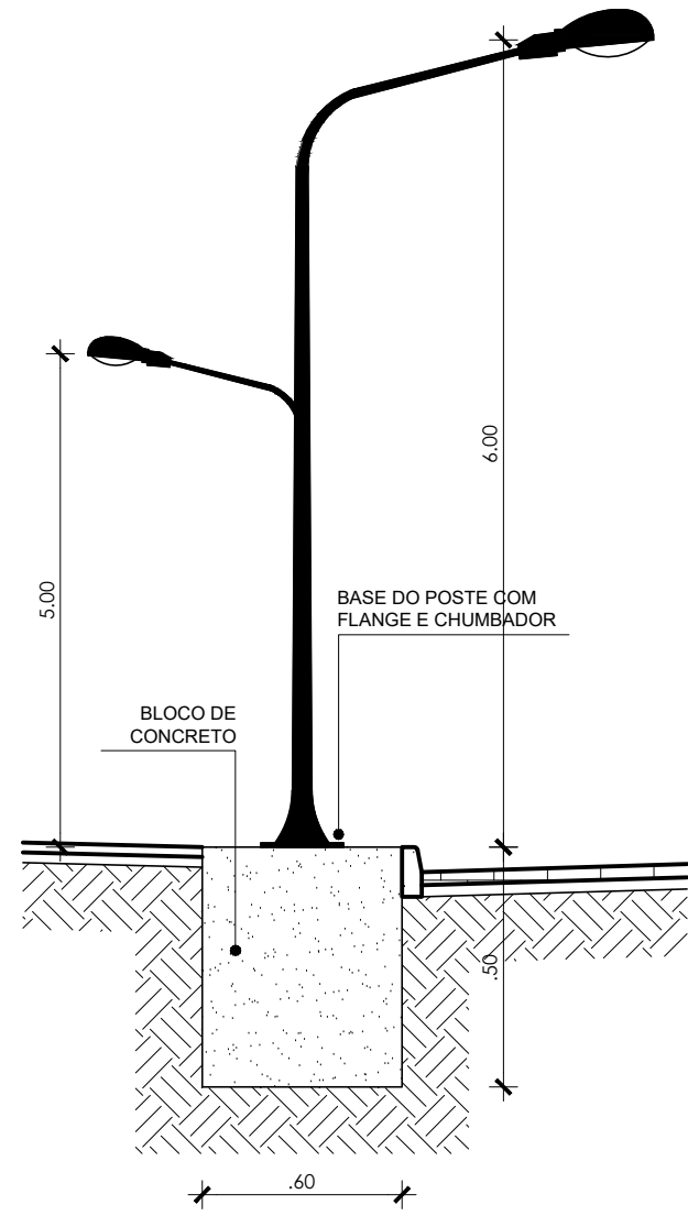
6 DETALHE TÍPICO - POSTE P/ ILUMINAÇÃO PÚBLICA SEM ESCALA
