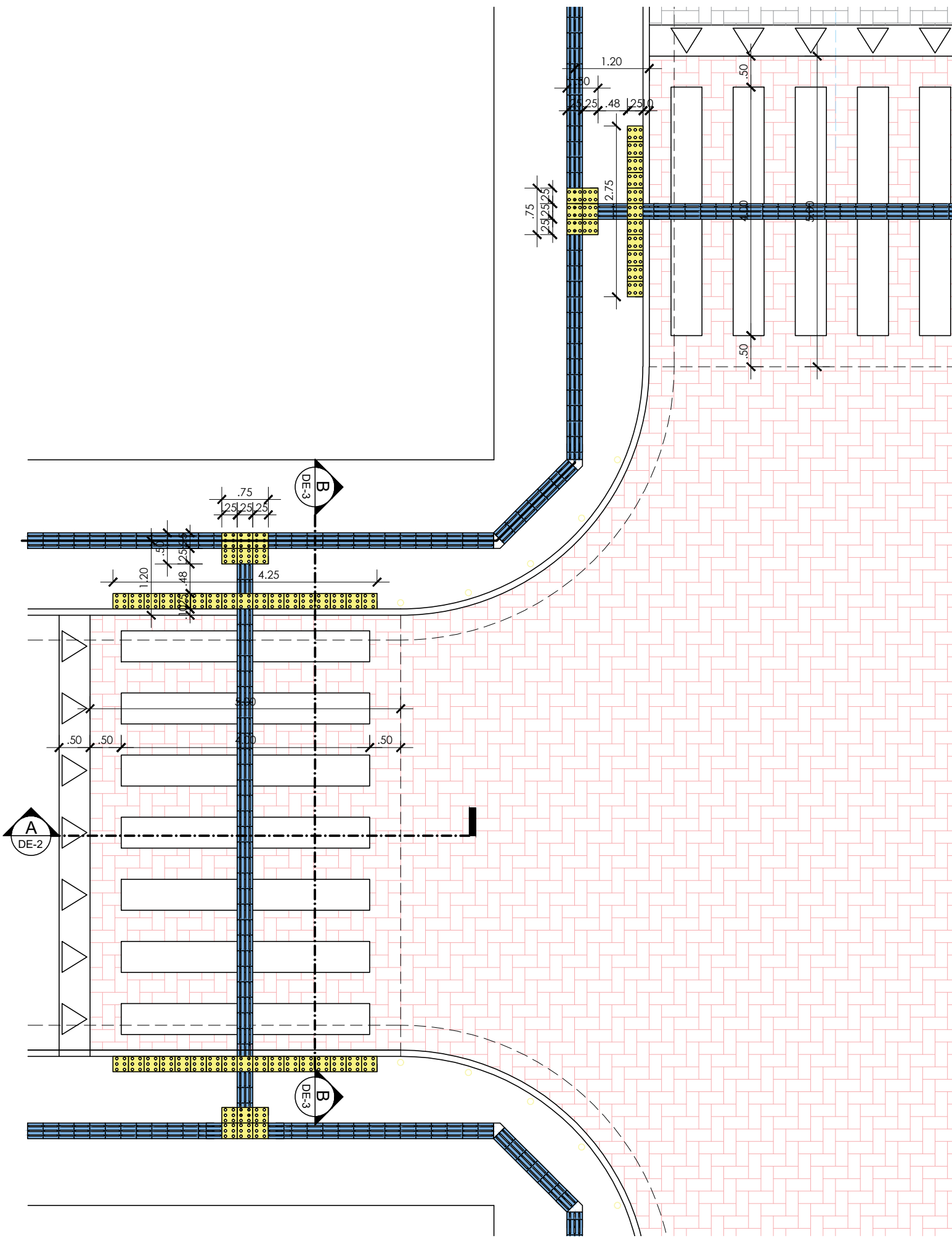
1 DETALHE TÍPICO - PISO TÁTIL E FAIXA ELEVADA ESCALA 1:75
