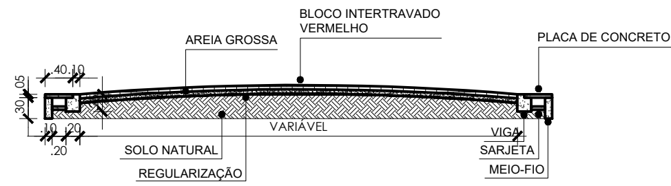
3 CORTE BB- FAIXA ELEVADA ESCALA 1:75
