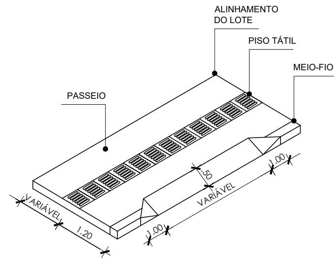
5 DETALHE TÍPICO - REBAIXO DE CALÇADA P/ ACESSO DE VEÍCULOS SEM ESCALA
