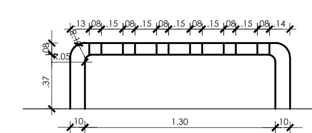
8 DETALHE TÍPICO - BANCO DE CONCRETO SEM ESCALA
