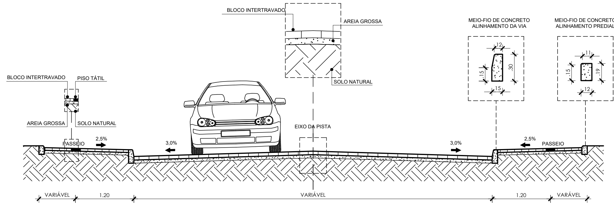
4 DETALHE TÍPICO - PISTA DE ROLAMENTO SEM ESCALA
