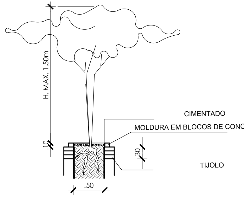
7 DETALHE TÍPICO - ÁRVORE SEM ESCALA
