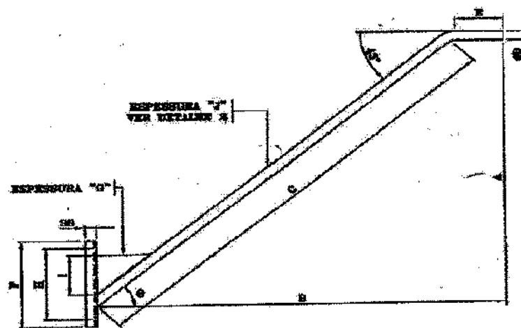
VISTA LATERAL
