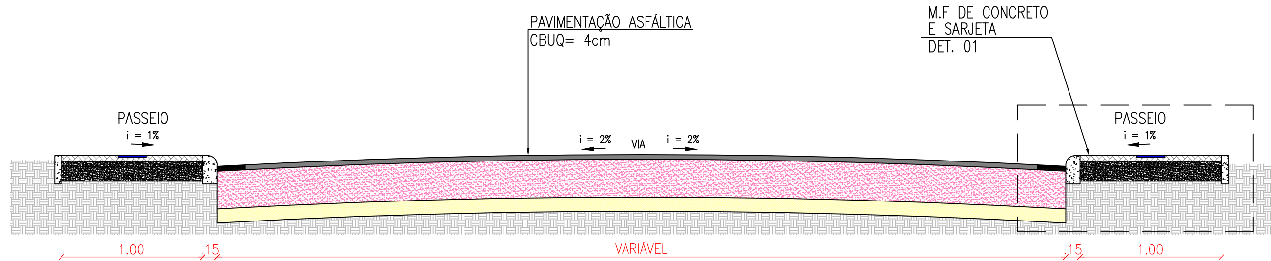
SEÇÃO TIPO
