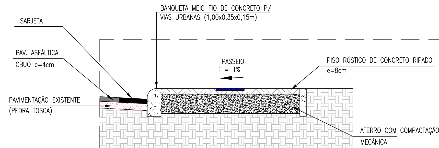
DETALHE MEIO FIO
