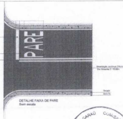
Faixa de Pare Curva Simples
