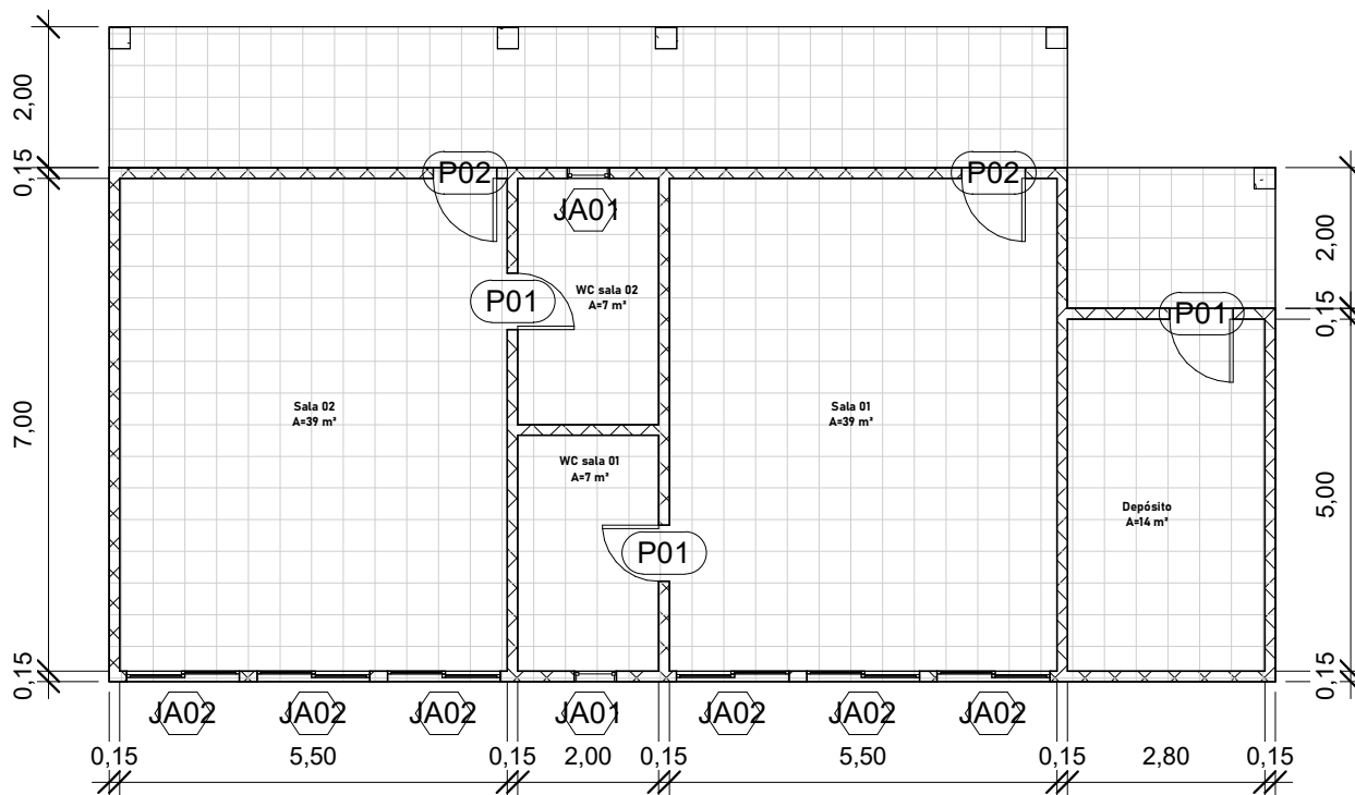
1 TÉRREO 1 : 100
