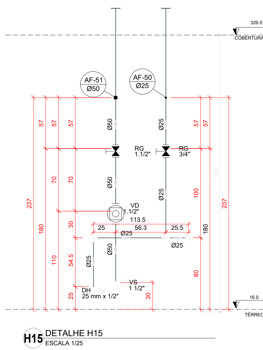
H15 DETALHE H15 ESCALA 1/25
