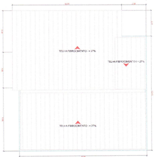
02 COBERTURA
