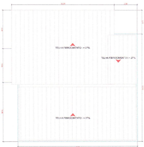
02 COBERTURA
