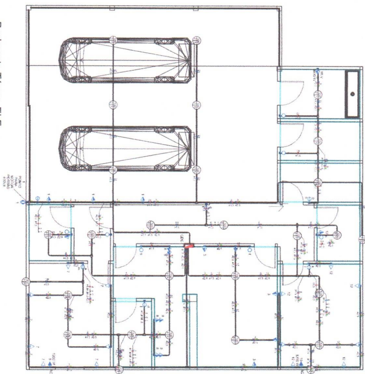
1 Pavimento Térreo-ELE 1 : 50
