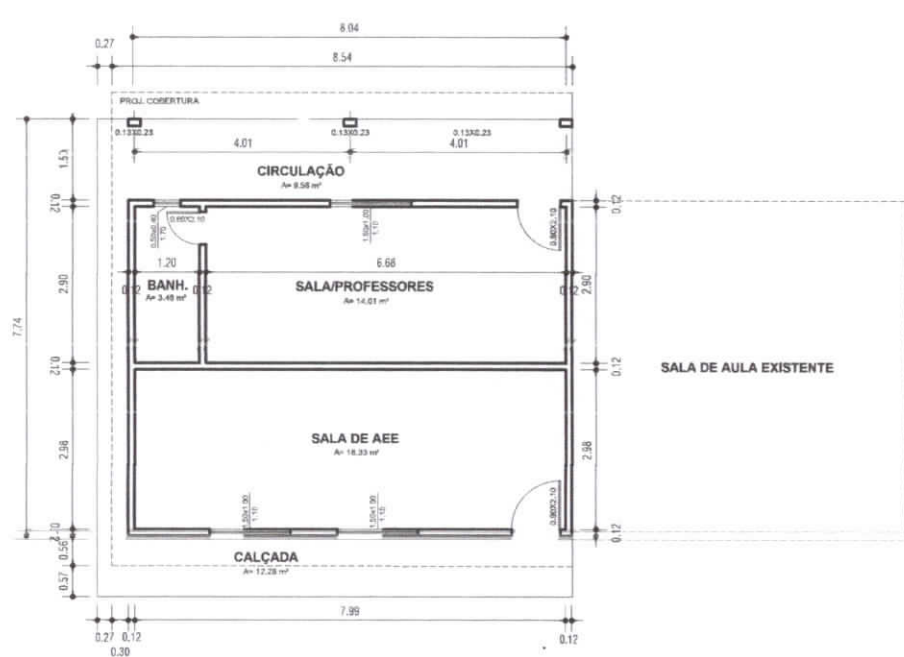
PLANTA BAIXA - E. M. E. F. SÃO PEDRO DA ÁGUA BRANCA - CONSTRUÇÃO DAS SALAS: AEE E PROFESSORES
