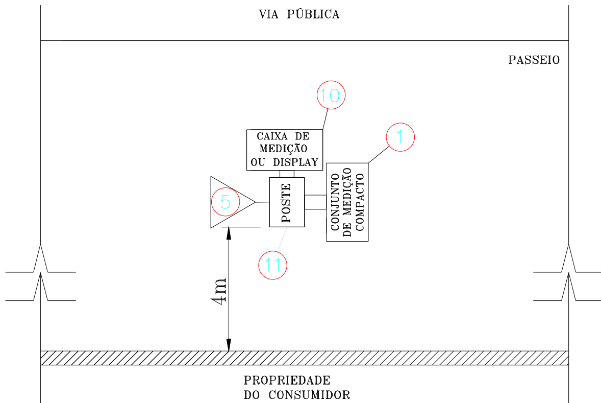
CONJUNTO COMPACTO CONJUNTO DE MEDIÇÃO COMPACTO E CAIXA DE MEDIÇÃO INSTALADO EM POSTE NO LIMITE DA VIA PÚBLICA
