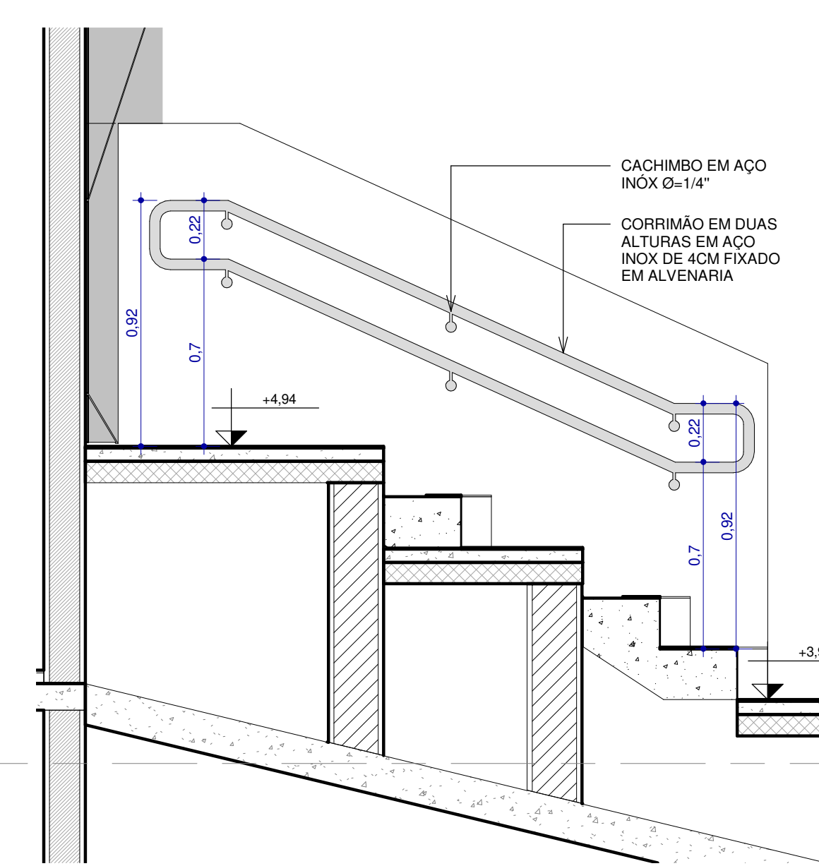
8 GUARDA CORPO 02 - CORTE 01 1 : 20
