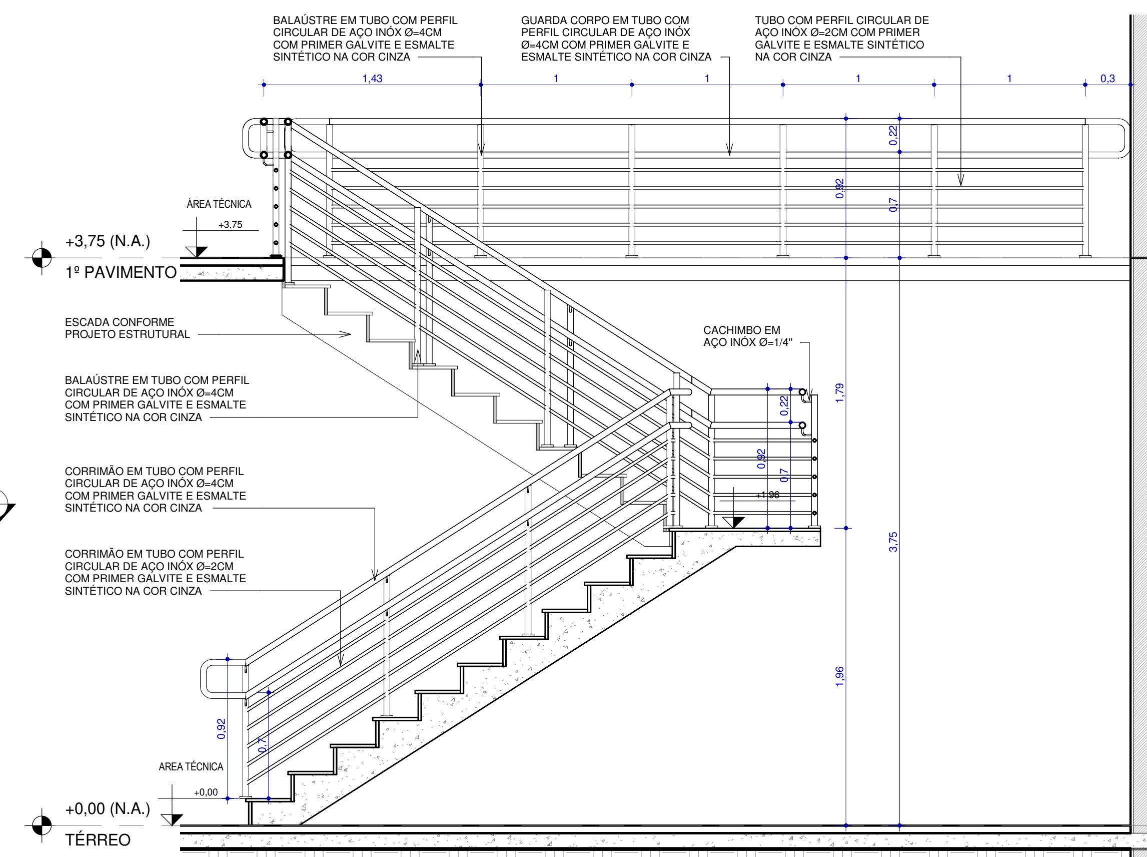
4 ESCADA 02 - CORTE 01 1 : 25
