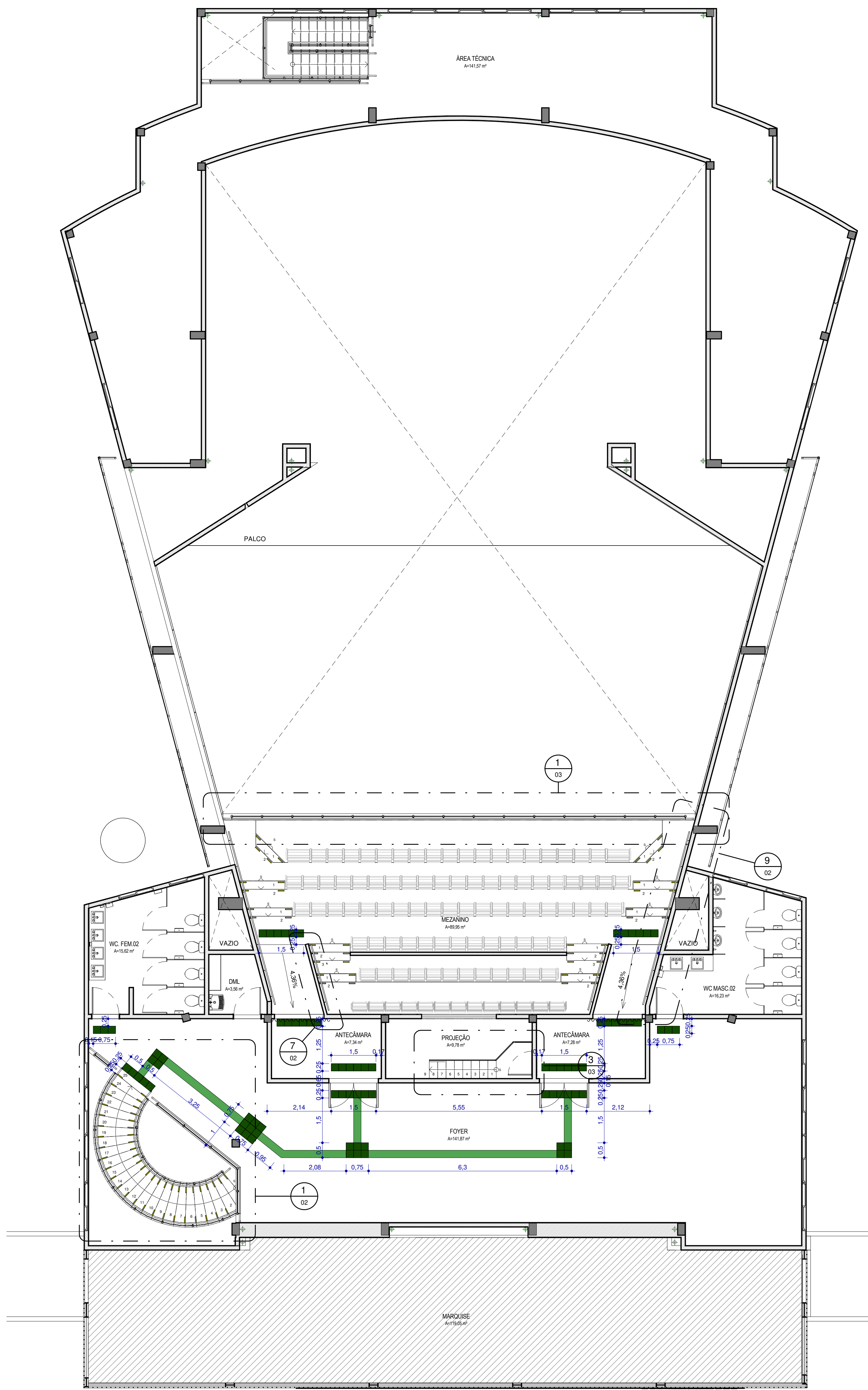
2 PLANTA DE ACESSIBILIDADE MEZANINO 1:75
