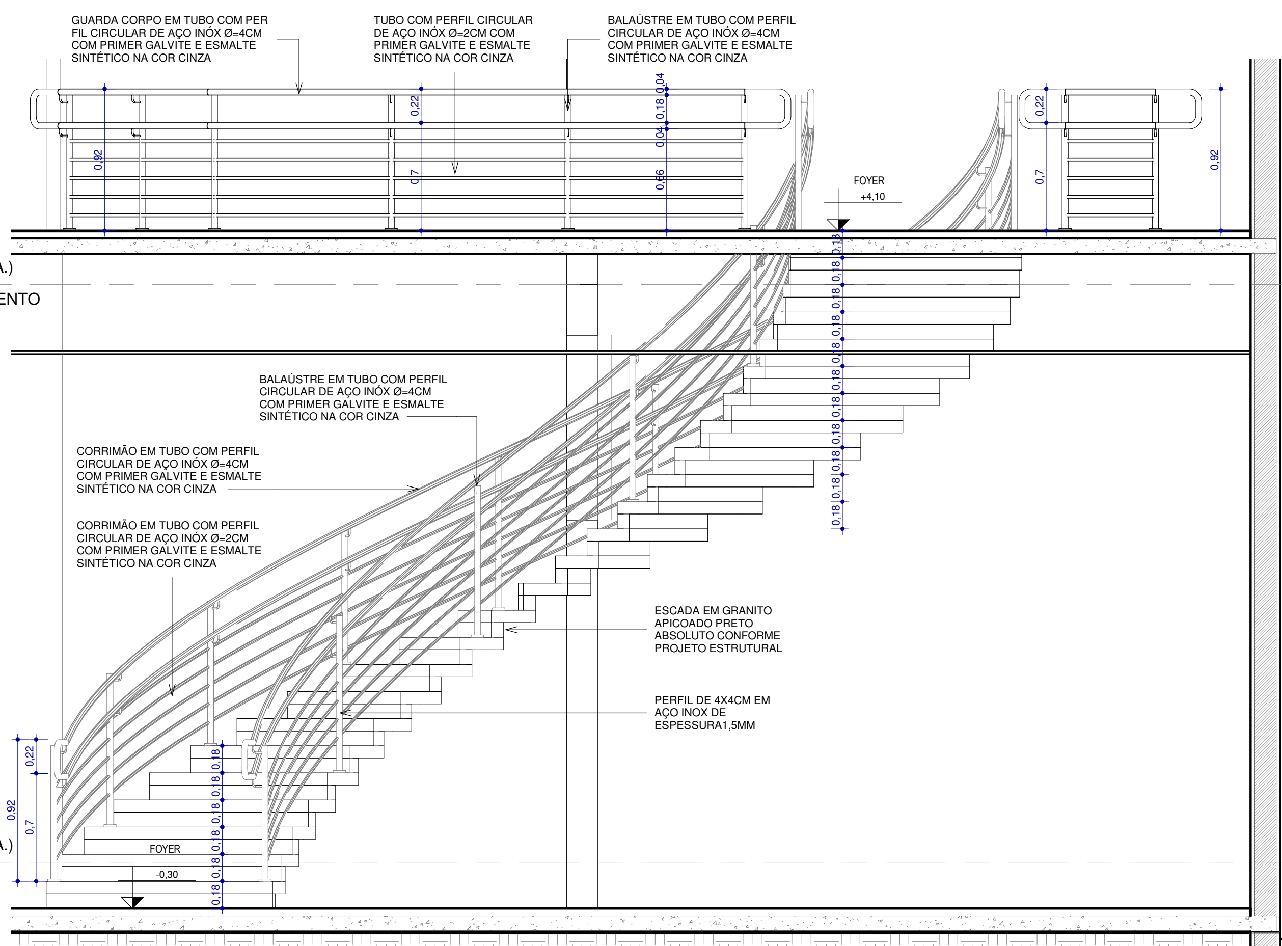
2 ESCADA 01 E GUARDA CORPO 01 - CORTE 01 1 : 25
