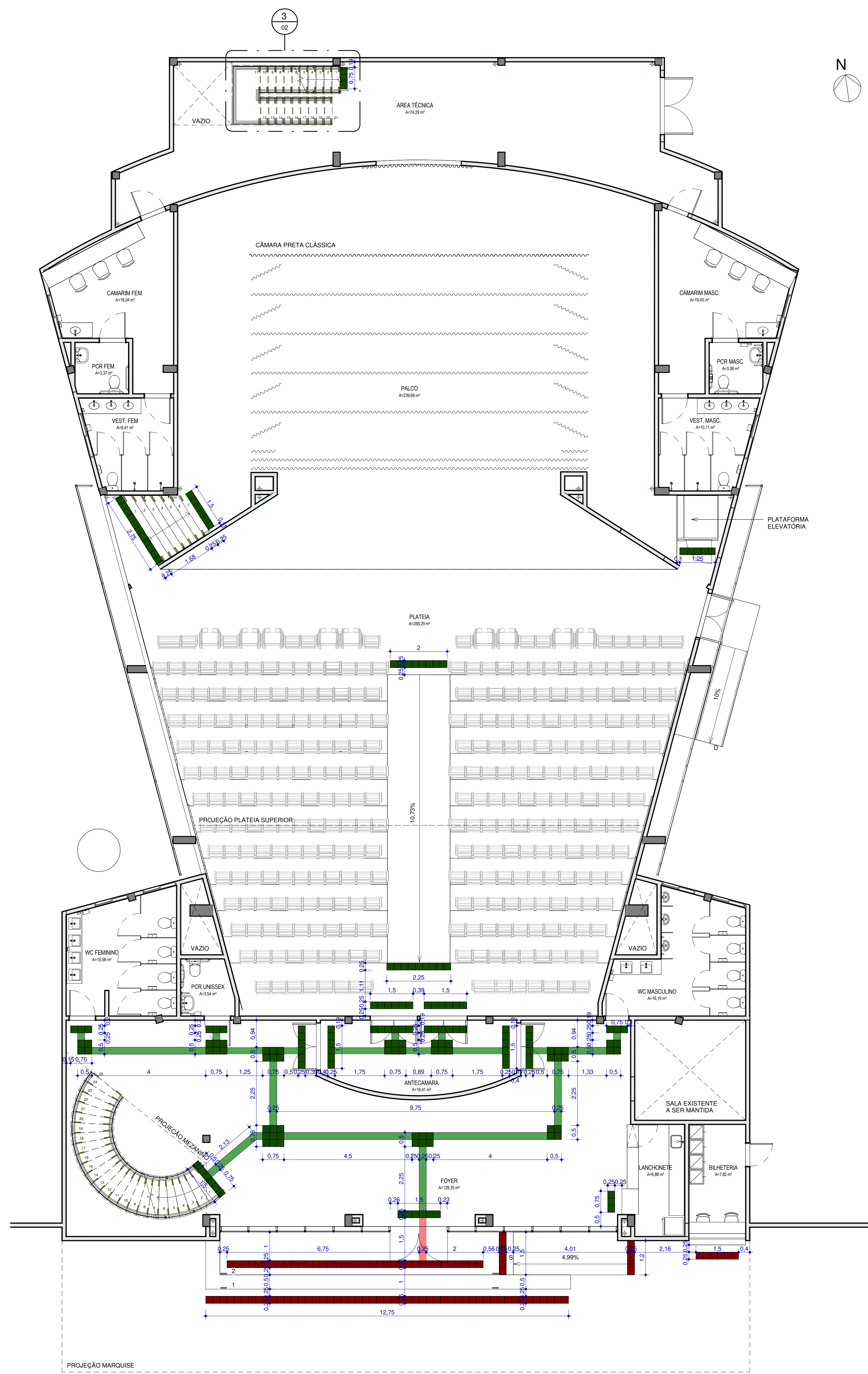
1 PLANTA DE ACESSIBILIDADE TÉRREO 1:75
