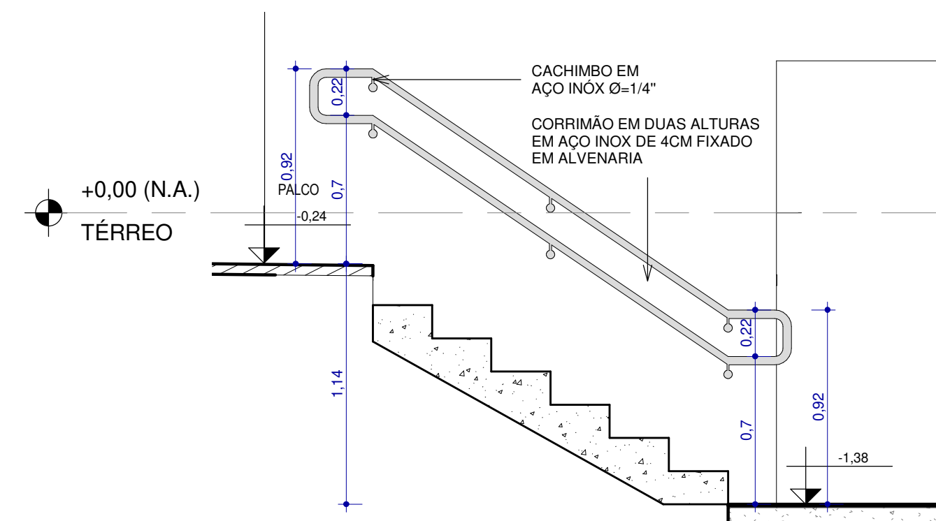
6 ESCADA 03 - CORTE 01 1 : 25
