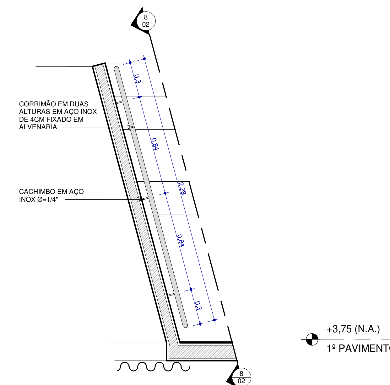
7 DET. GUARDA CORPO 02 1 : 20
