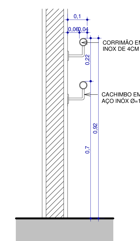
13 DET. CORRIMÃO TIPO 02 1 : 10
