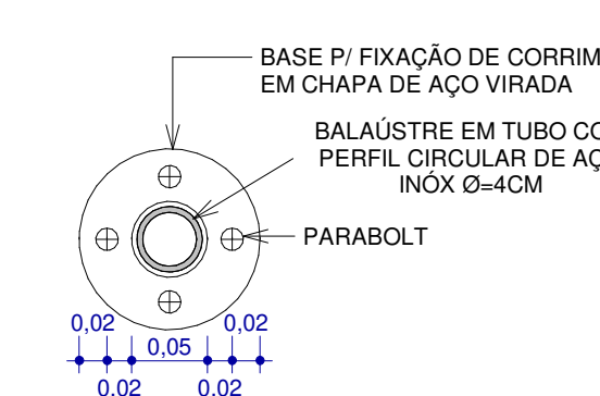
12 FIXAÇÃO CORRIMÃO TIPO 01 1 : 5
