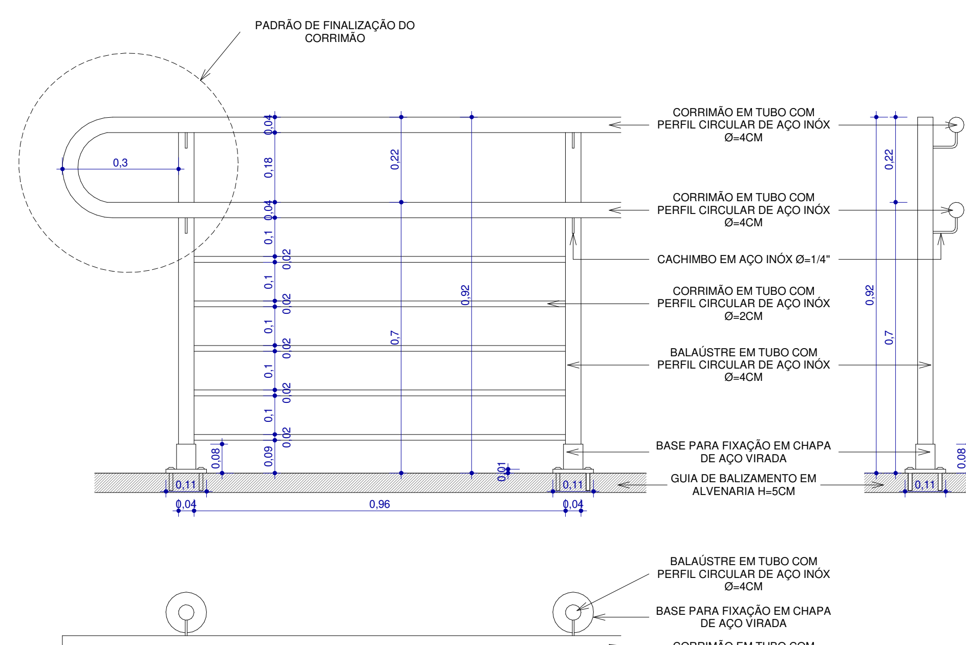
11 DET. CORRIMÃO TIPO 01 1 : 10
