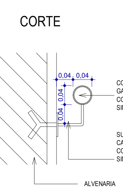
14 DETALHE EMPUNHADORA 1 : 5
