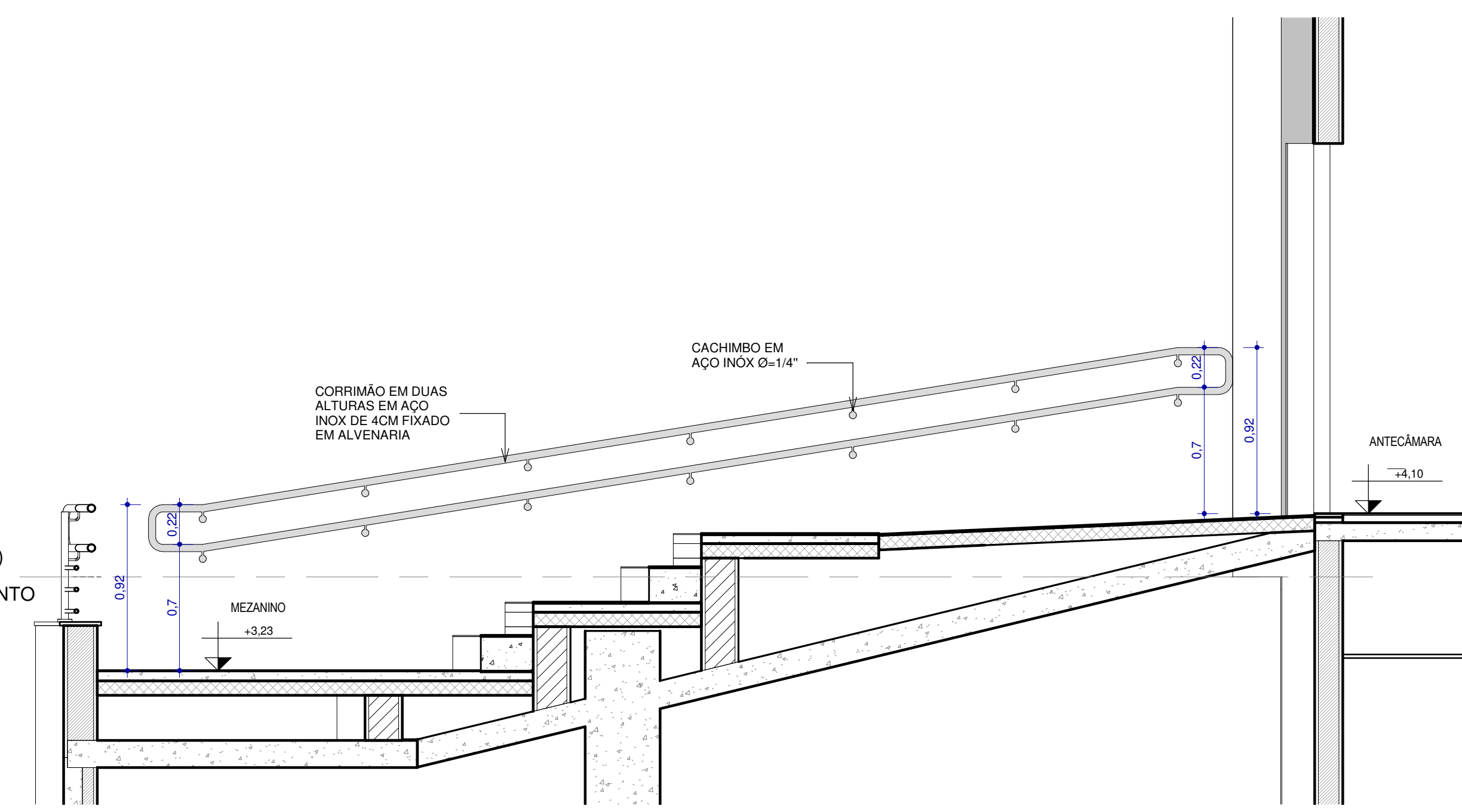
10 GUARDA CORPO 03 - CORTE 01 1 : 25
