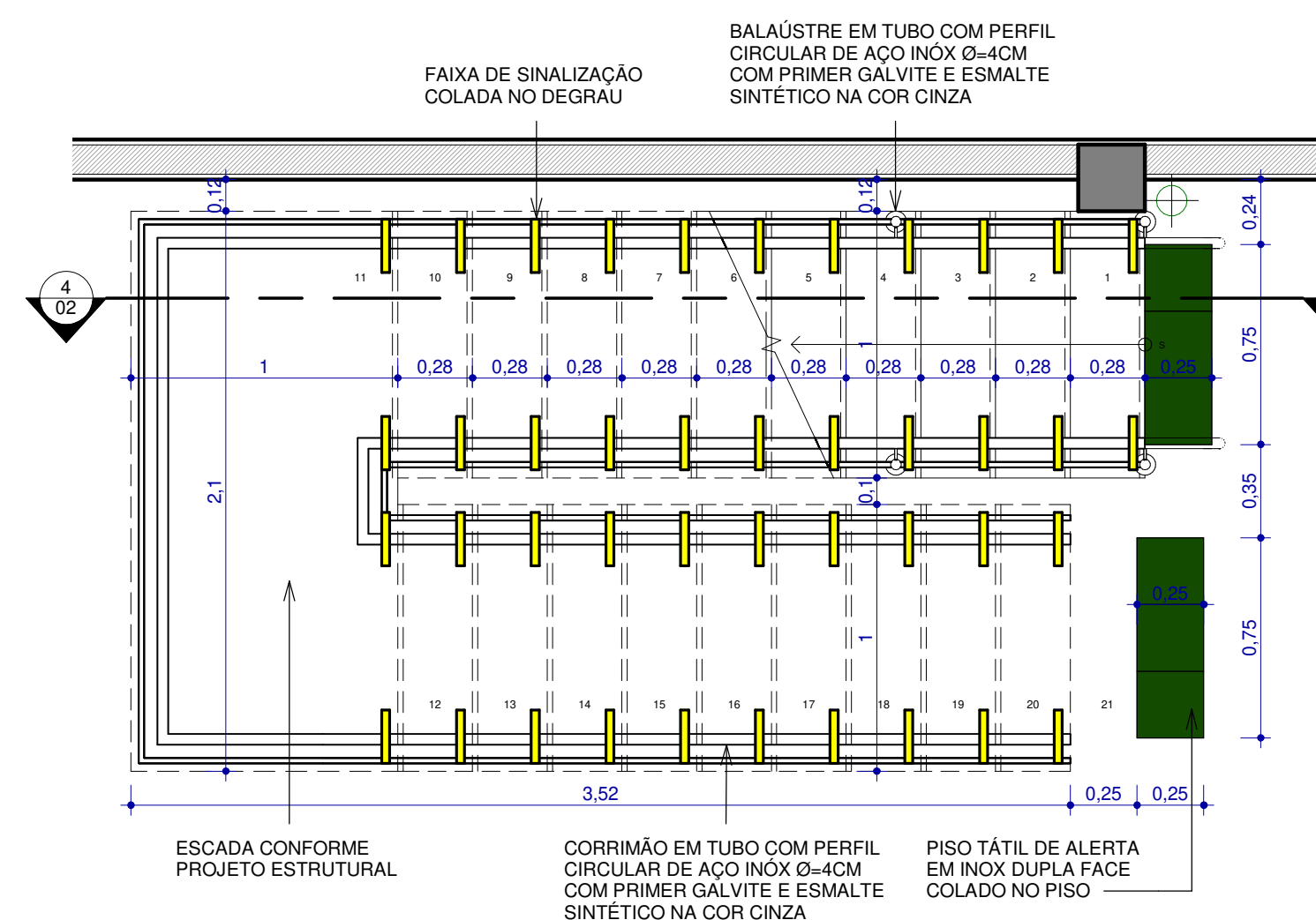
3 DET. ESCADA 02 1 : 25
