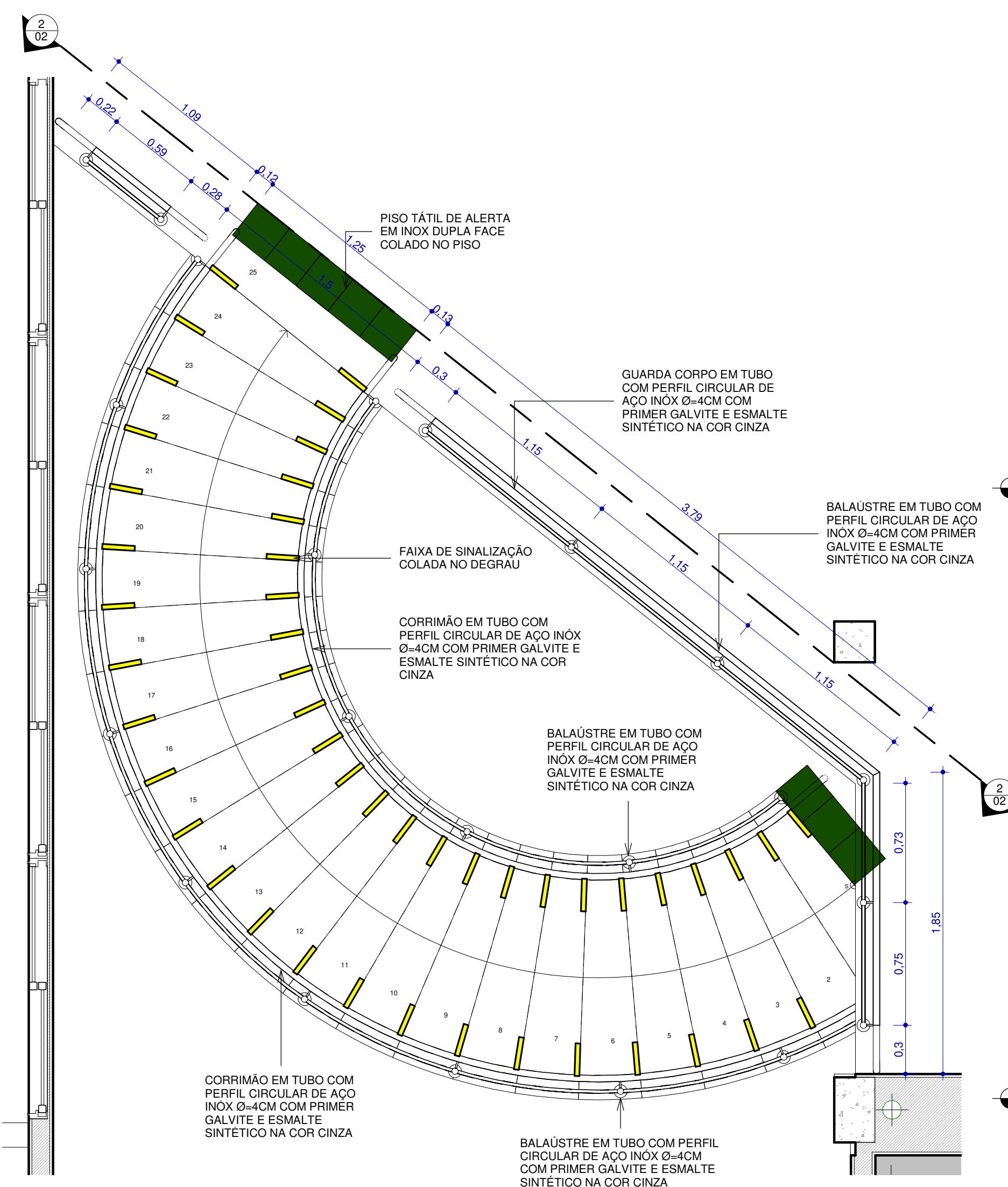
1 DET. ESCADA 01 E GUARDA CORPO 01 1 : 25
