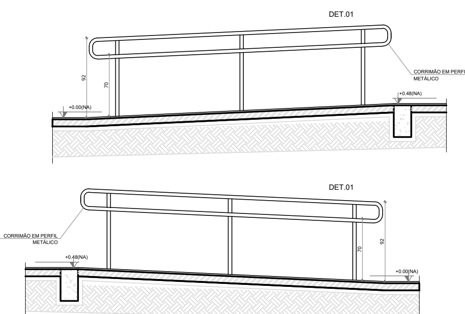
RAMPA ENTRADA esc S/E
