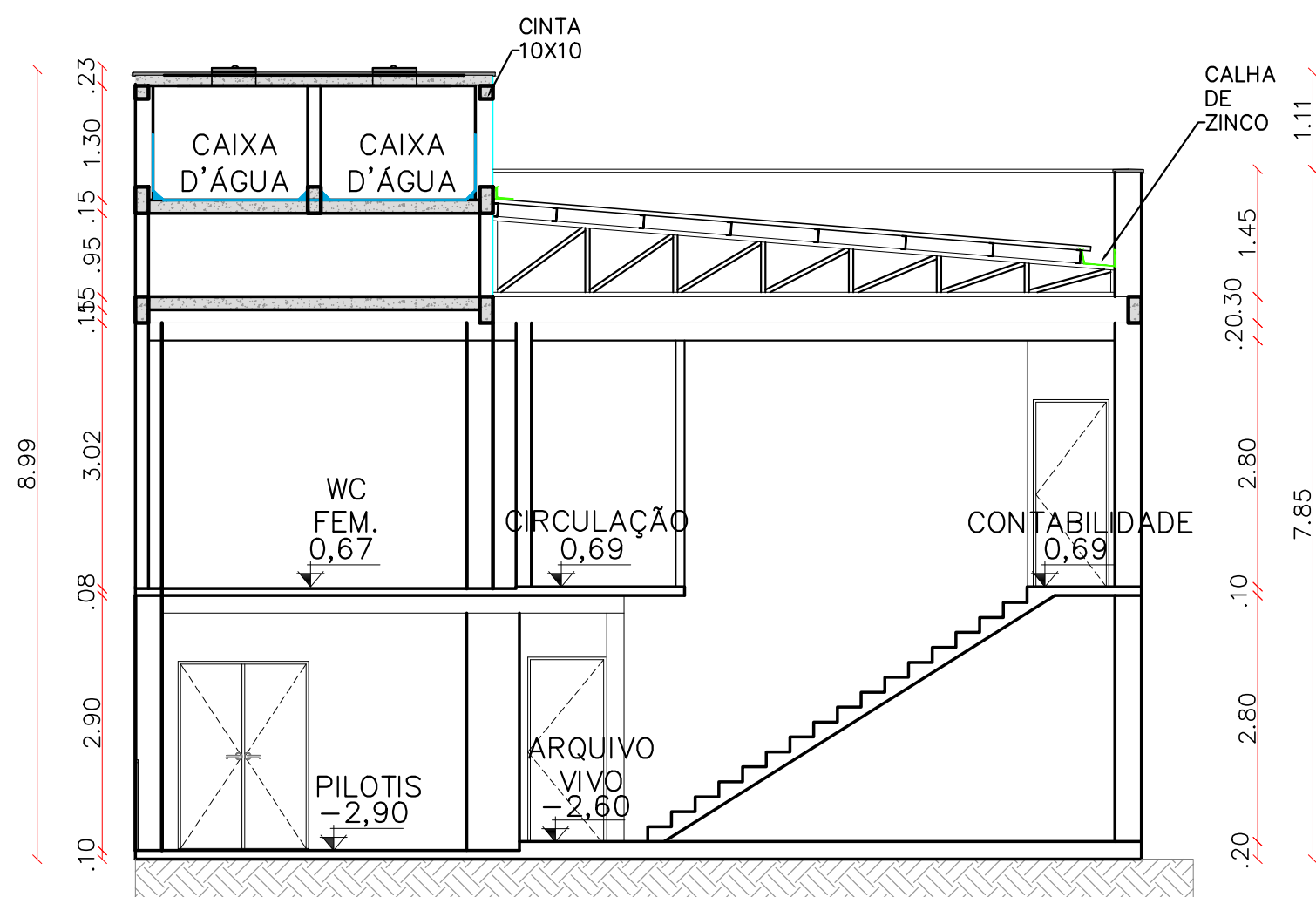
CORTE B esc 1:75
