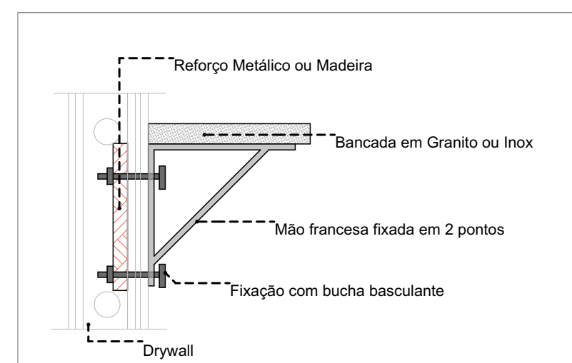
DETALHE 01: REFORÇO EM DRYWALL Escala:1:20
