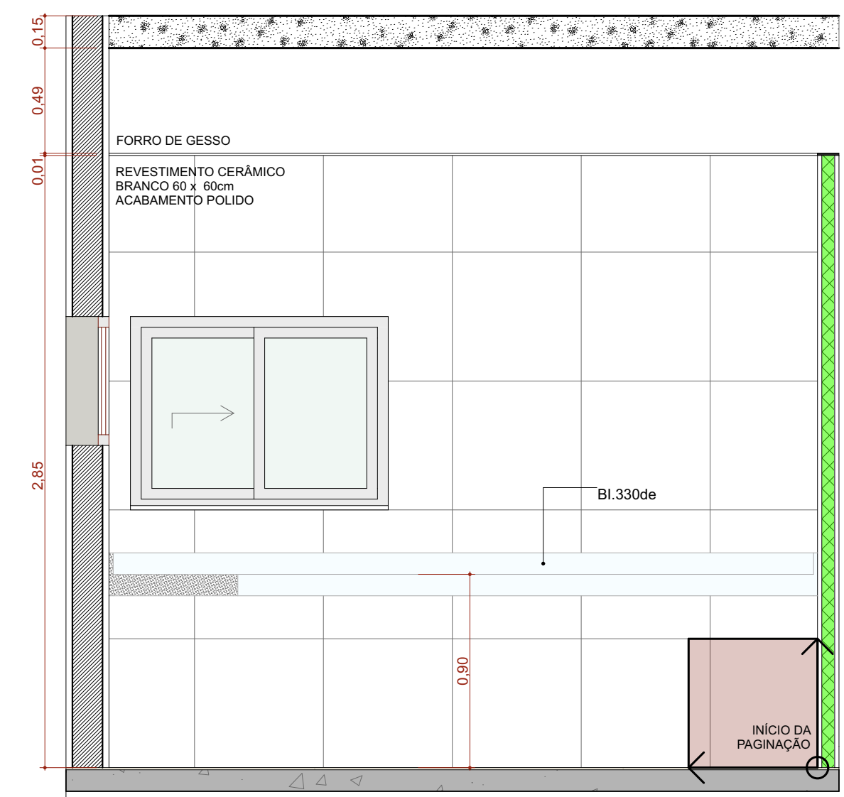
A.M.06 VISTA 3 Escala: 1:25
