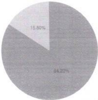
Curva ABC
