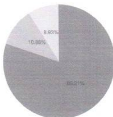
Curva ABC
