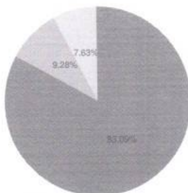
Curva ABC
