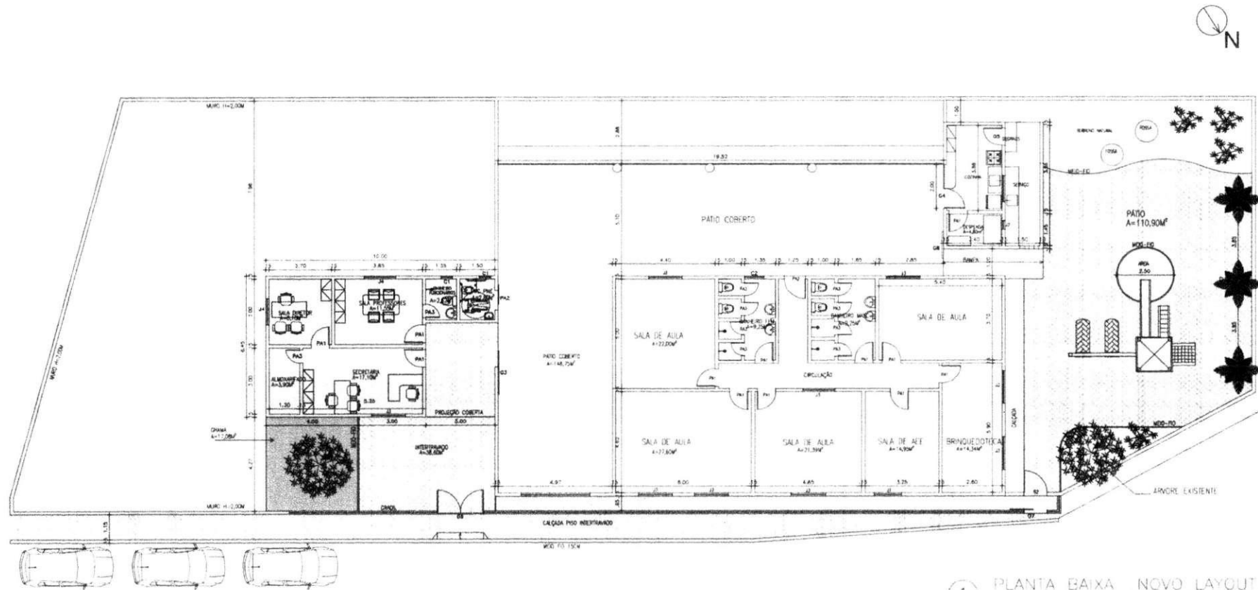
1 PLANTA BAIXA NOVO LAYOUT ESC. 1:100
