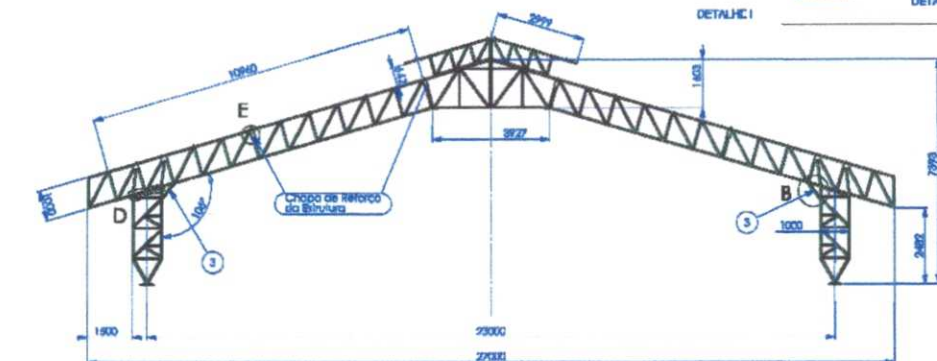
3 PÓRTICO PÓRTICO QG - A SEM ESCALA
