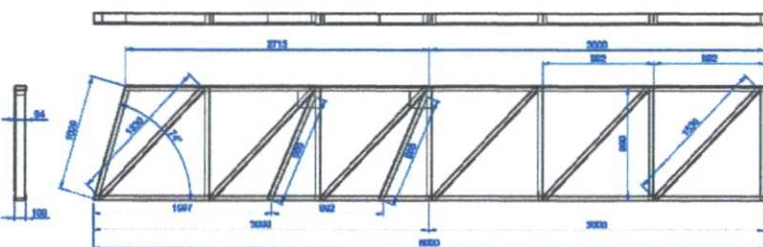
2 TESSOURA APOIO NA COLUMA TESSOURA DE - B SEM ESCALA
