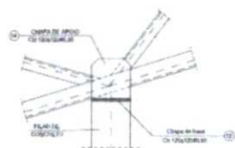
7 DETALHE B ESCALA 1/10
