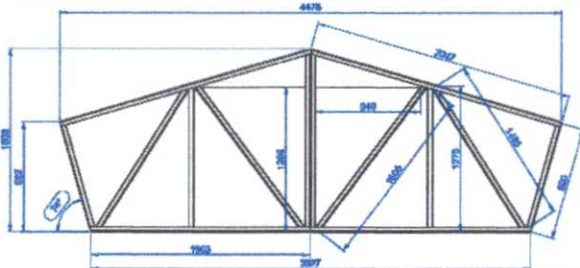
3 CAPELA UNIÃO TREFILADA CAPELA DE - A SEM ESCALA
