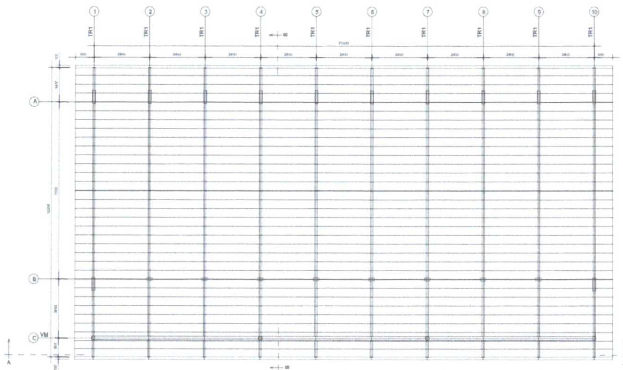
1 ESQUEMA GERAL DA ESTRUTURA ESCALA 1/75
