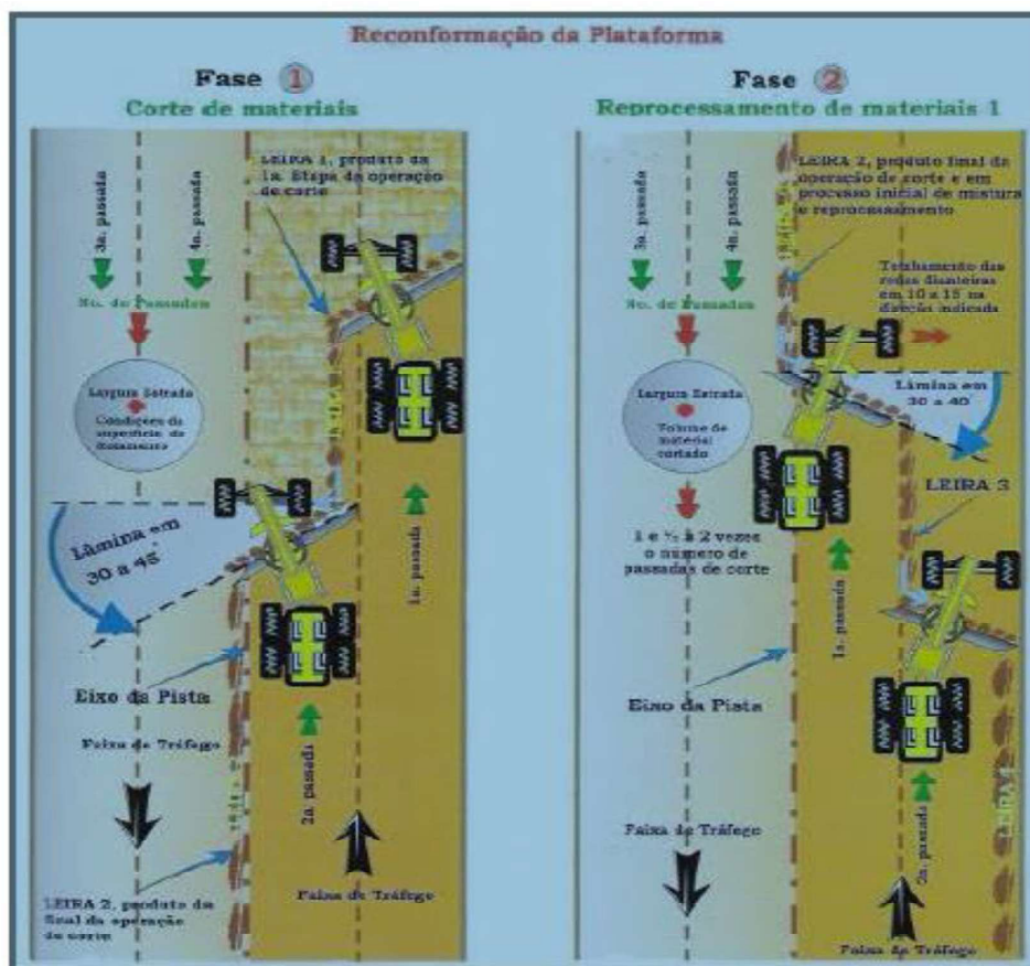
FASE 01 E 02 – PROCESSO DE REGULARIZAÇÃO DO TERRENO NATURAL
