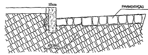
03 PERFIL TRANSVERSAL ESCALA = 1:50
