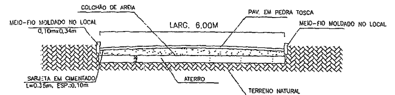
03 PERFIL TRANSVERSAL ESCALA = 50M
