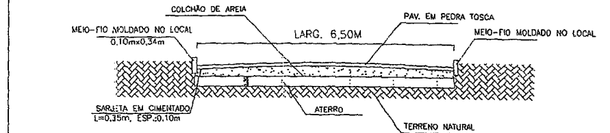
03 PERFIL TRANSVERSAL ESCALA = 1:500
