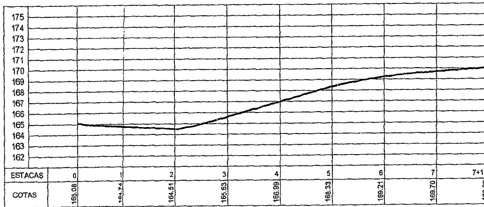
02 PERFIL LONGITUDINAL ESCALA = 1:500
