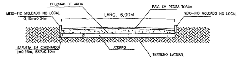
03 PERFIL TRANSVERSAL ESCALA - 50M
