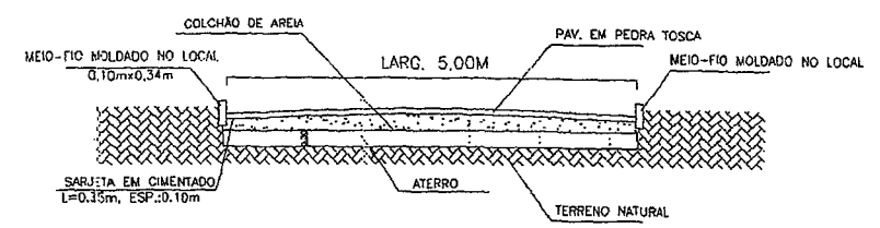
03 PERFIL TRANSVERSAL ESCALA = 1:50
