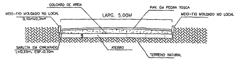
03 PERFIL TRANSVERSAL ESCALA = 1:50
