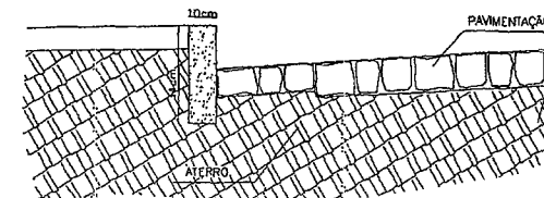
03 PERFIL TRANSVERSAL ESCALA - 50M
