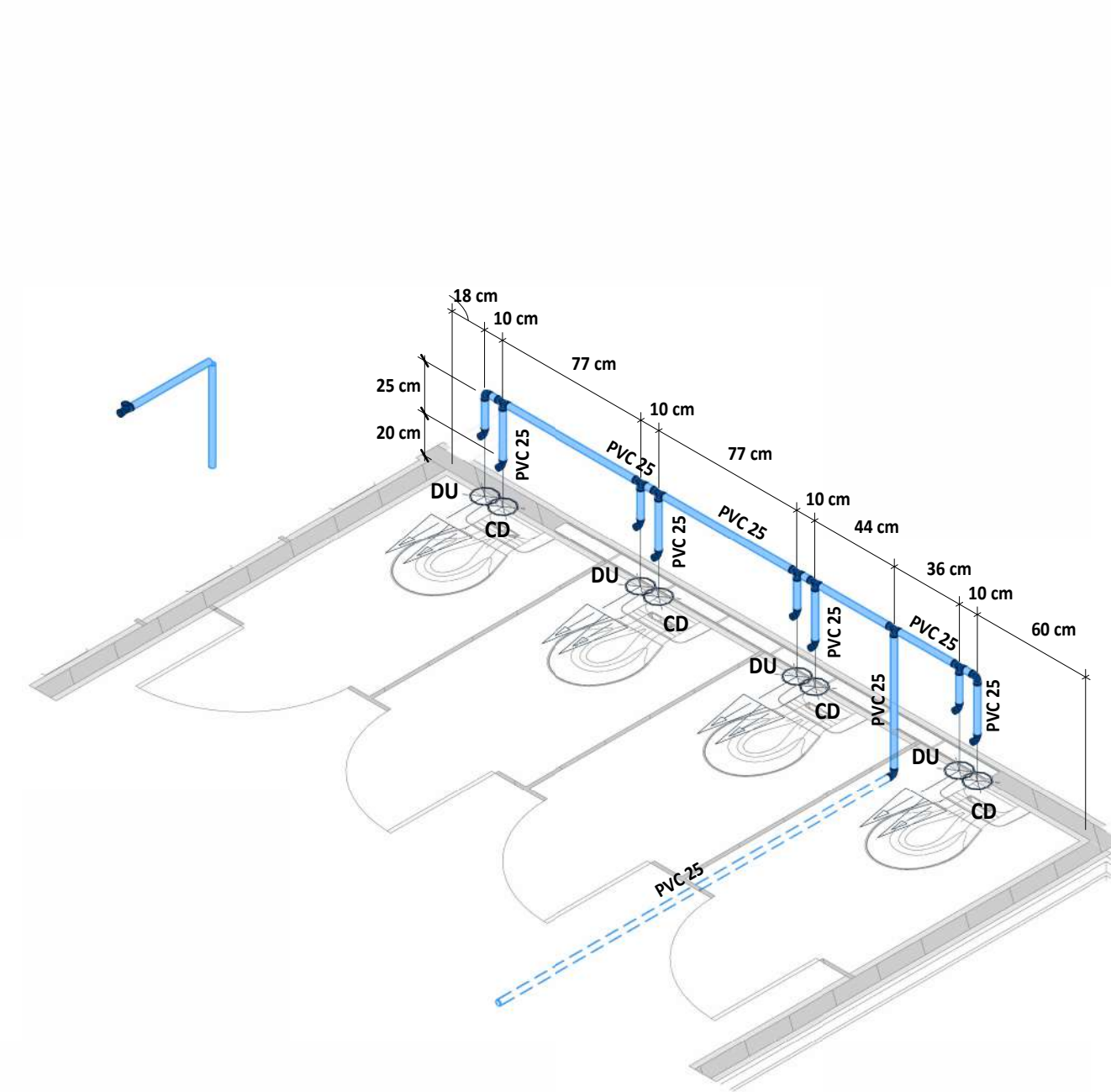
3 ISOMETRICO HID - DET 05 SEM ESCALA
