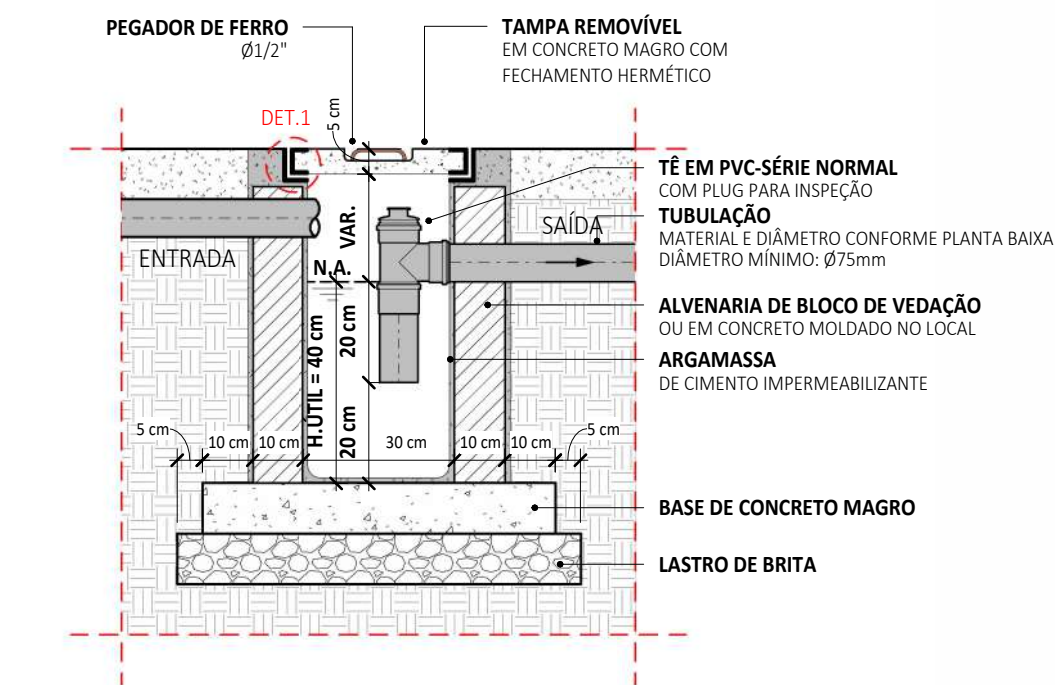
5 DET. 04 - CAIXA DE SABÃO/GORDURA (CGP) 1:15
