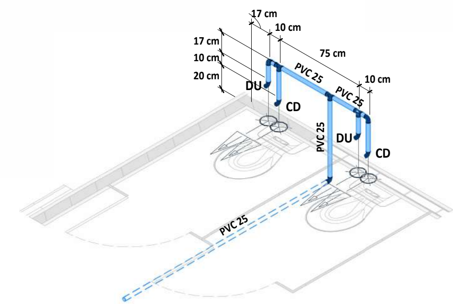
5 ISOMETRICO HID - DET 03 SEM ESCALA
