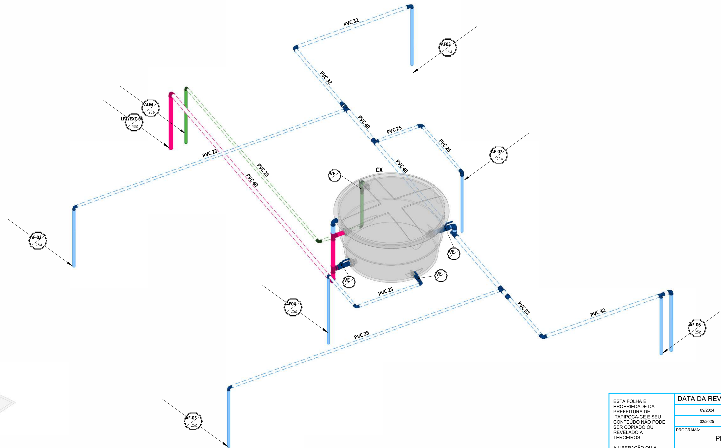
7 ISOMETRICO HID - DET 08 SEM ESCALA
