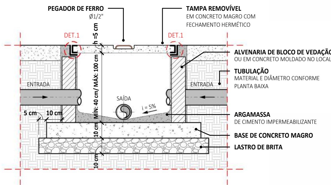
2 DET. 01 - CAIXA DE INSPEÇÃO (CI) SEM ESCALA
