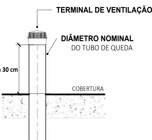
4 DET. 03 - TERMINAL DE VENTILAÇÃO 1:50
