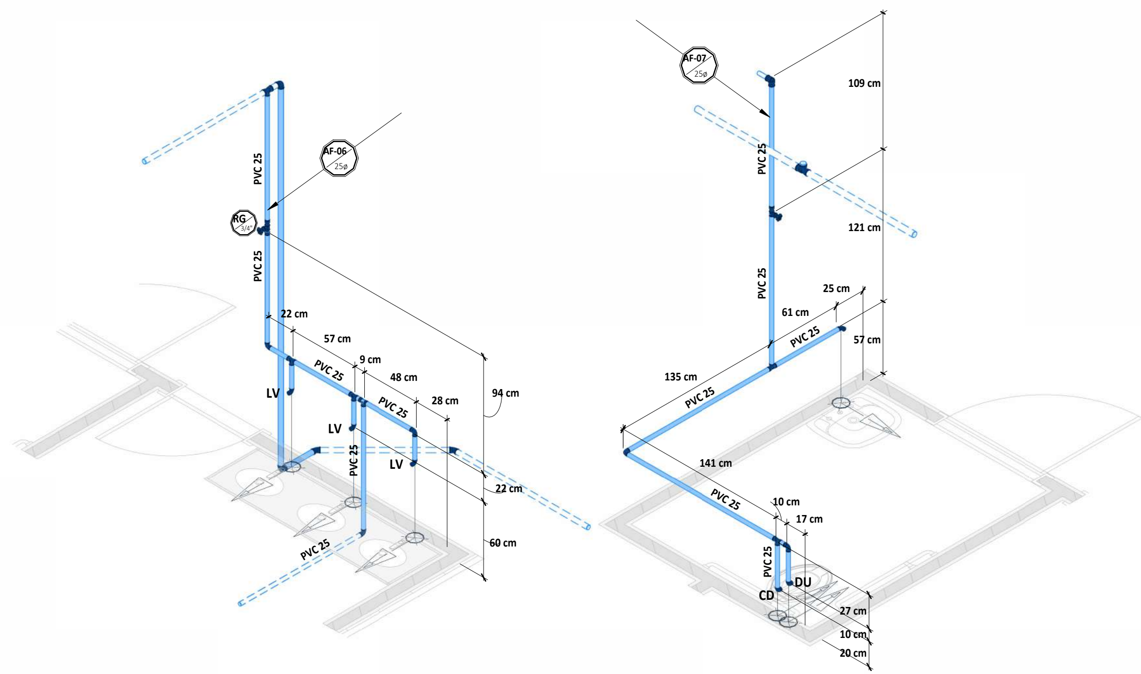
1 ISOMETRICO HID - DET 02 SEM ESCALA
