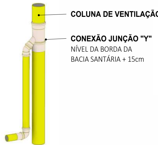
3 DET. 02 - COLUNA DE VENTILAÇÃO 1:50
