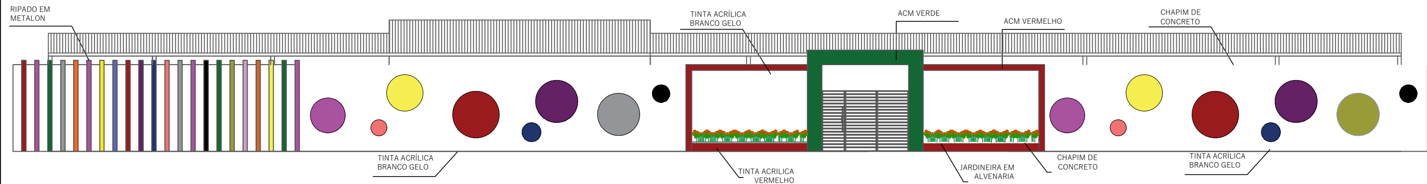
FACHADA DO MURO esc 1:75
