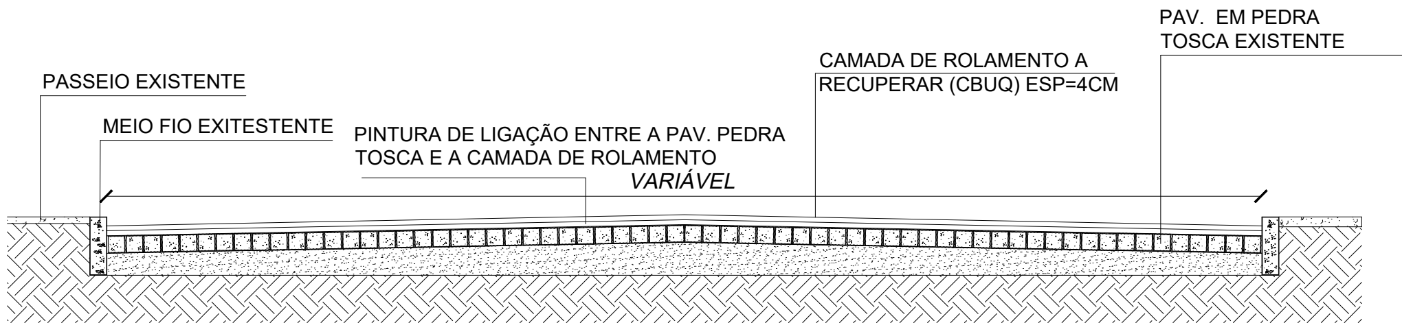
04 DETALHES DO CAP. ASFÁLTICO SEM ESCALA
