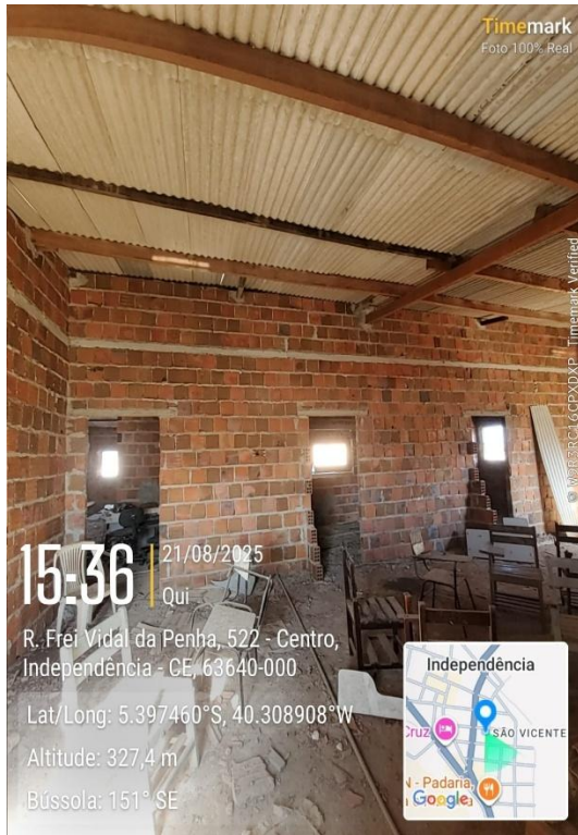
Foto 29 e 30: Paredes de alvenária, piso necessidade regularização
