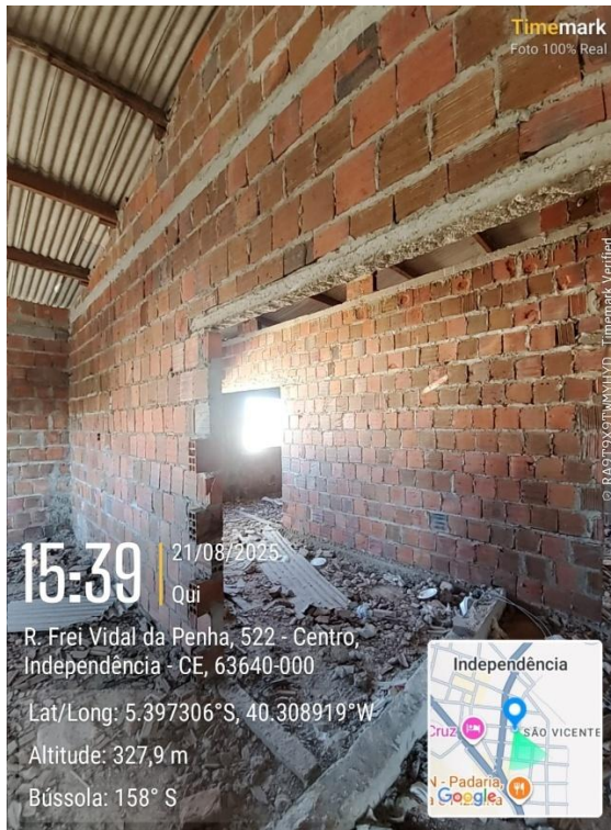
Foto 27 e 28: Paredes de alvenária, piso necessidade regularização
