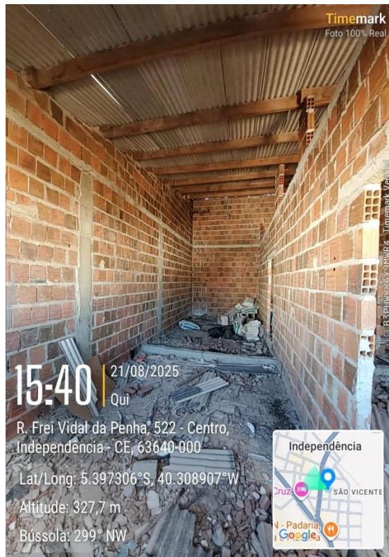
Foto 24 e 25: Paredes de alvenária, piso necessidade regularização, viga invertida aparente
