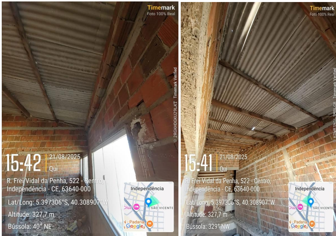
Foto 19 e 20: Cobertura com madeiramento e telha de fibrocimento.
