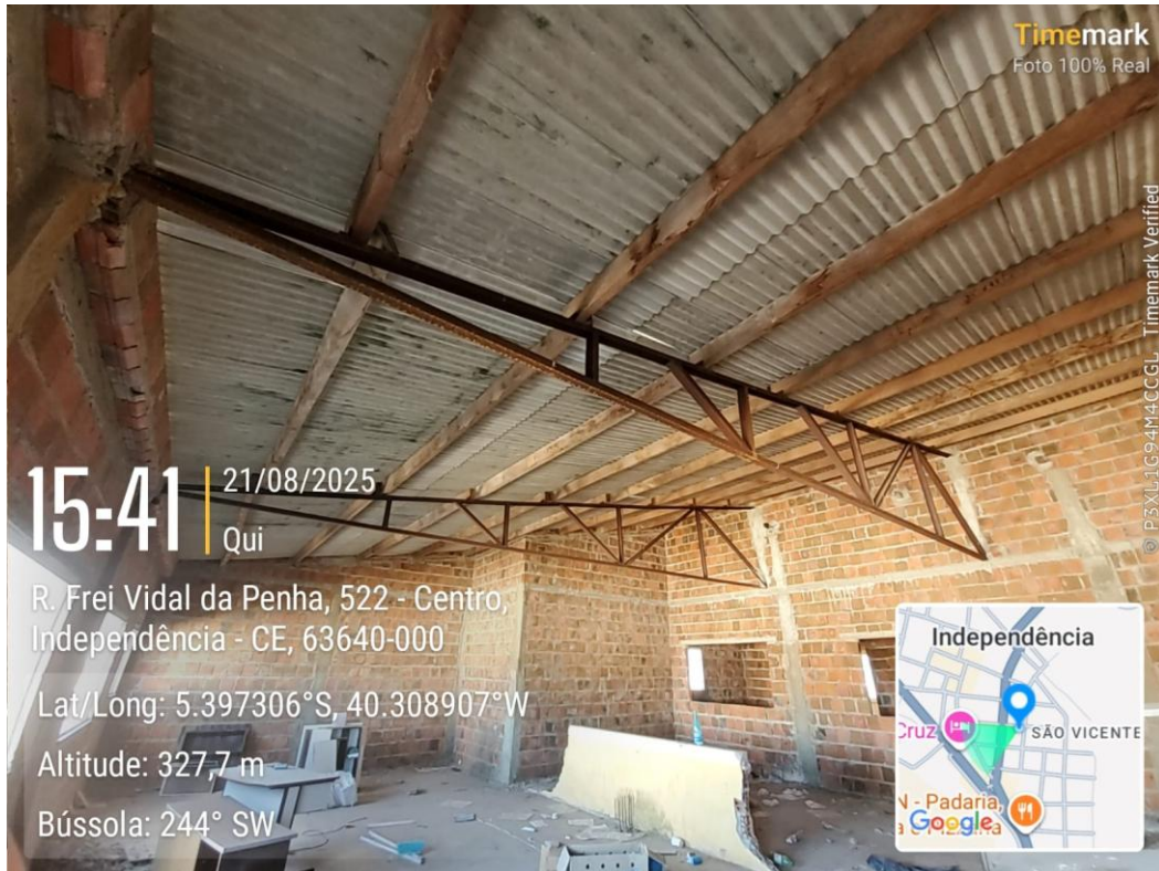
Foto 21: Cobertura parcialmente em estrutura metálica, madeiramento e telha de fibrocimento.
