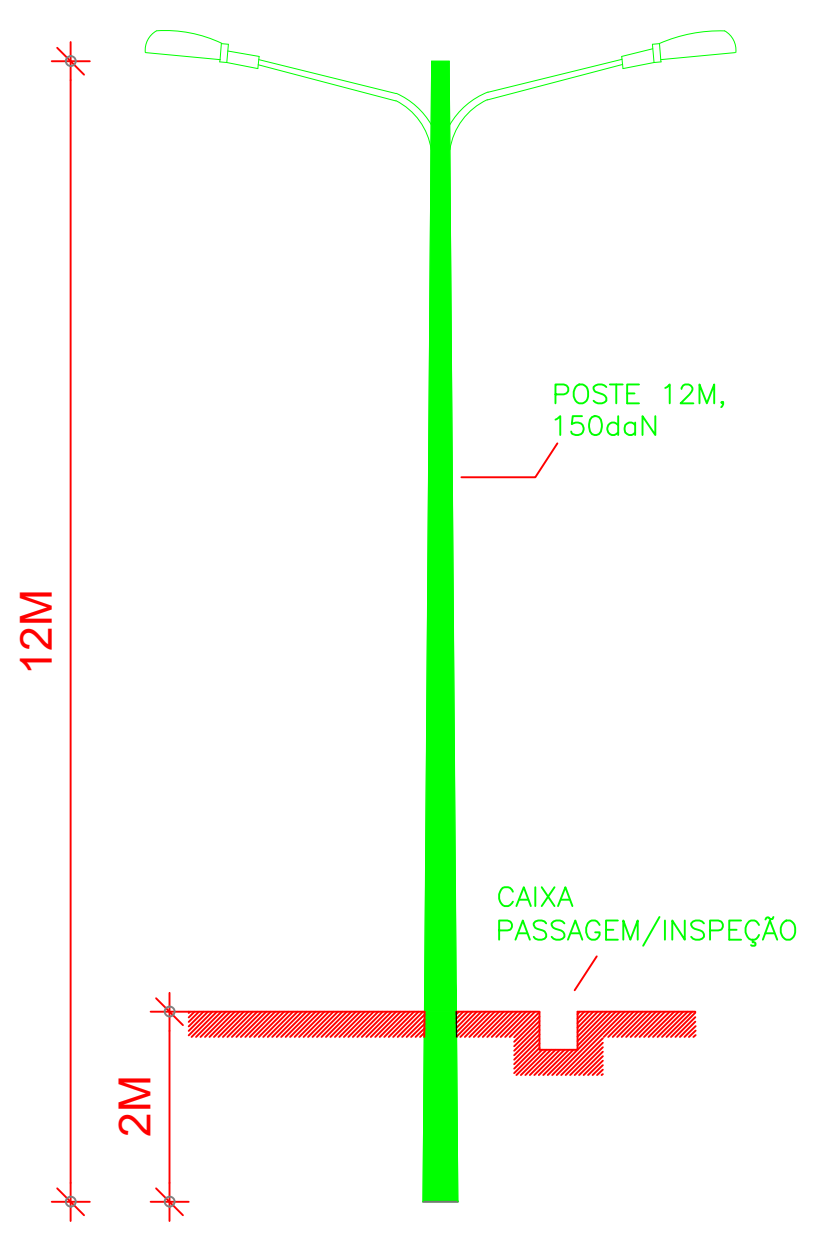
08 DETALHE POSTE SEM ESCALA
