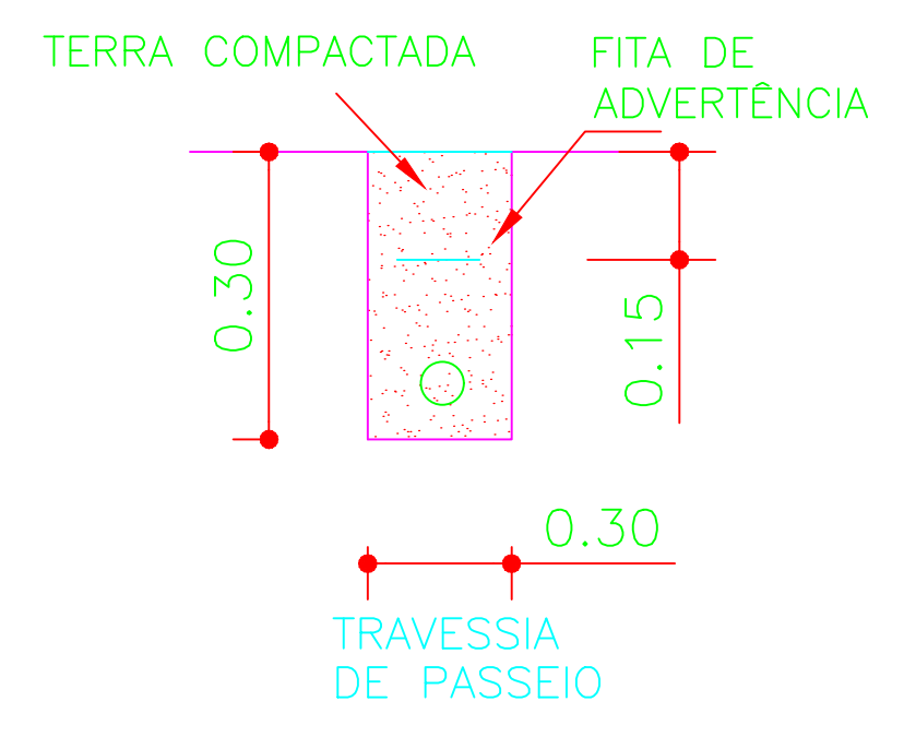
06 DETALHE DE TRAVESSIA SEM ESCALA
