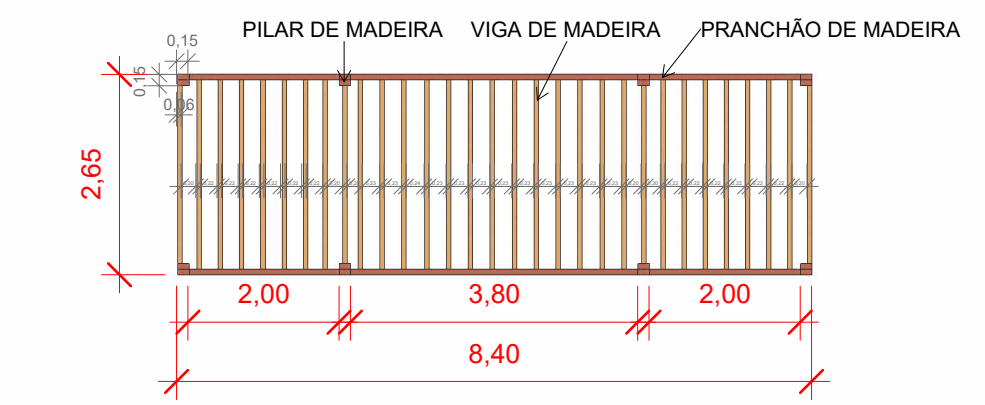
P PERGOLADO 1: 100
