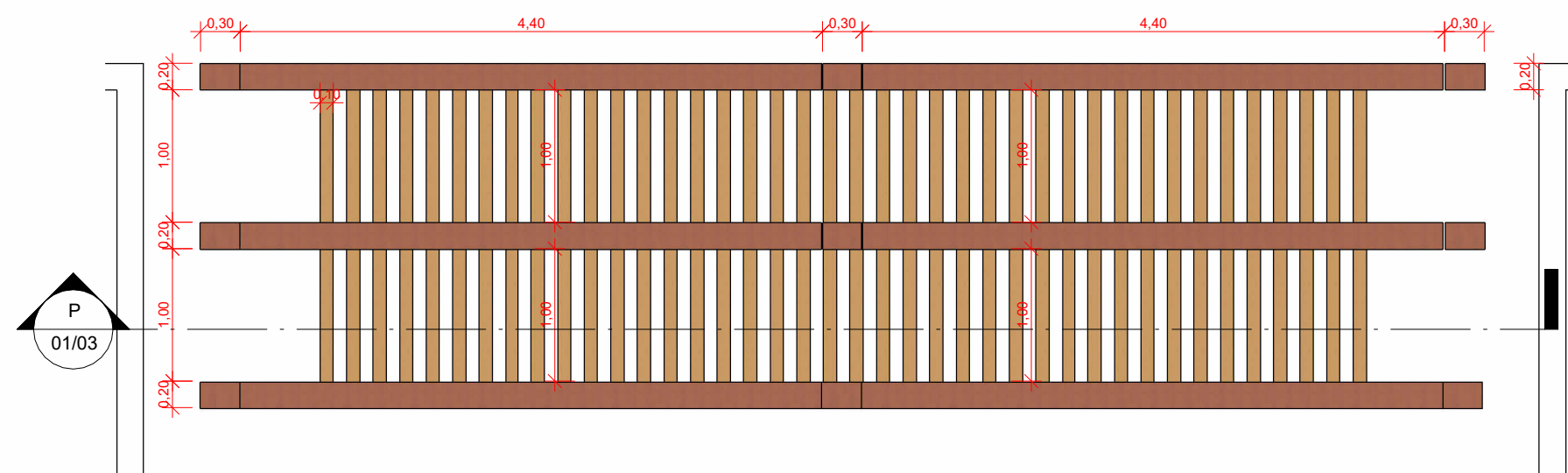
DETALHAMENTO PÓRTICO
