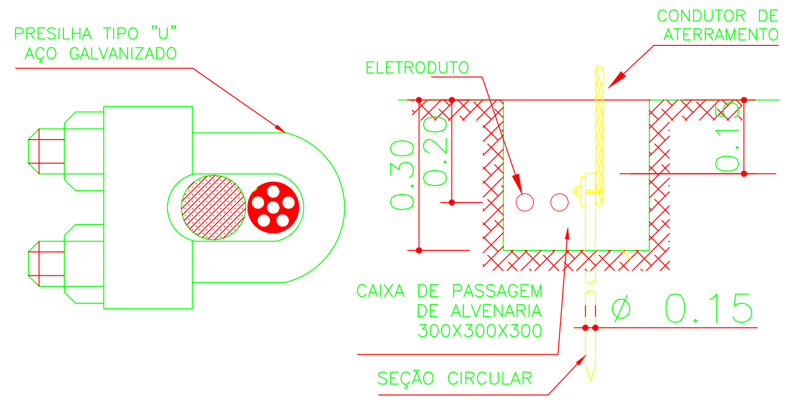
07 DETALHE DE ATERRAMENTO SEM ESCALA
