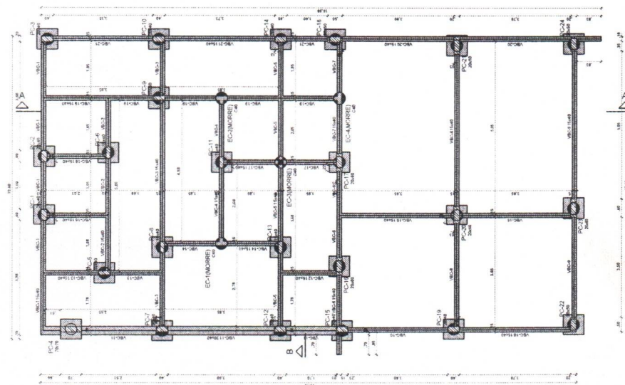
1 FORMA FUNDAÇÃO ESCM A 1/50
