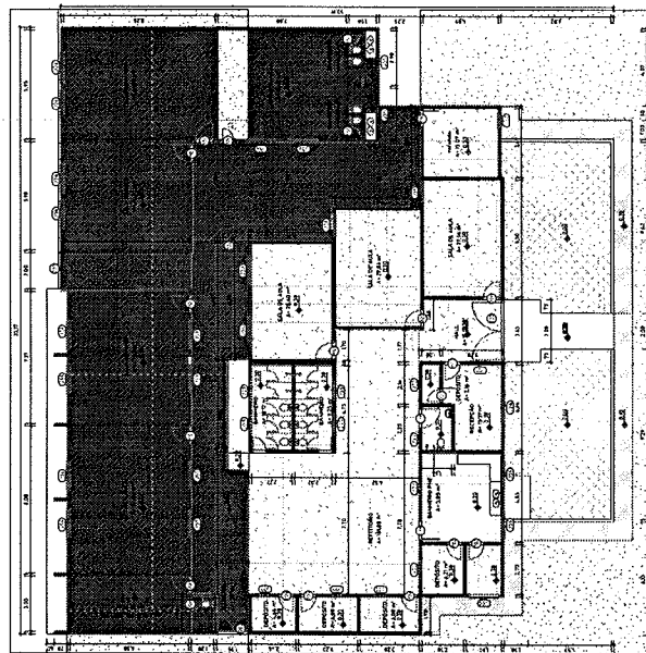
3 PLANTA BAIXA REFORMA - CONSTRUÇÃO
