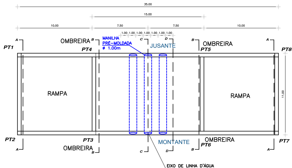
PLANTA BAIXA
