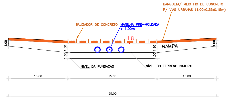
CORTE LONGITUDINAL
