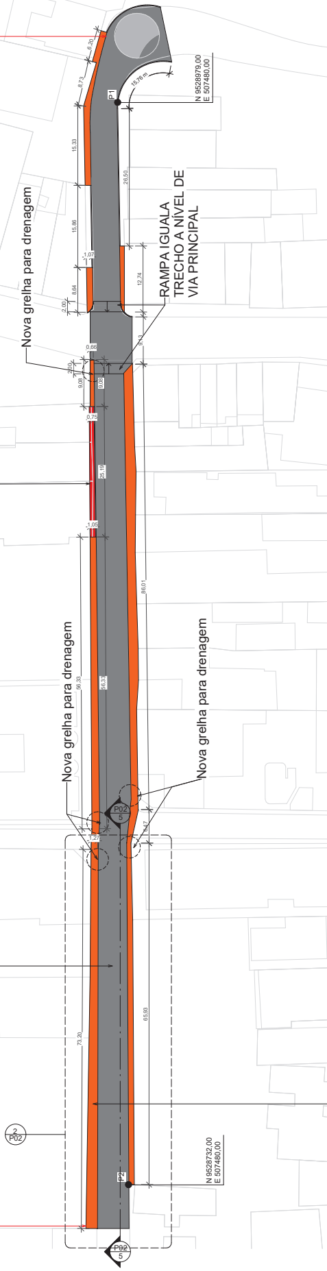
1 ESCALA 1:500 PAVIMENTAÇÃO JÚLIO HOLANDA - SITUAÇÃO DEPOIS
