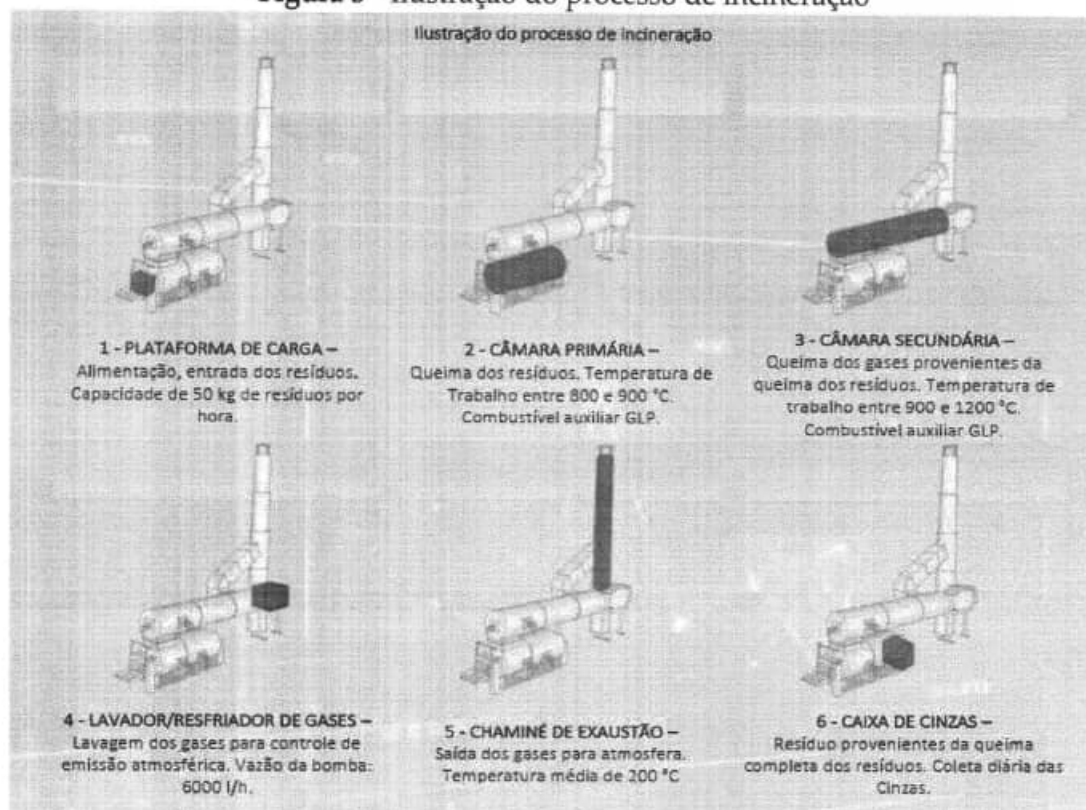
Figura 3 - Ilustração do processo de incineração
