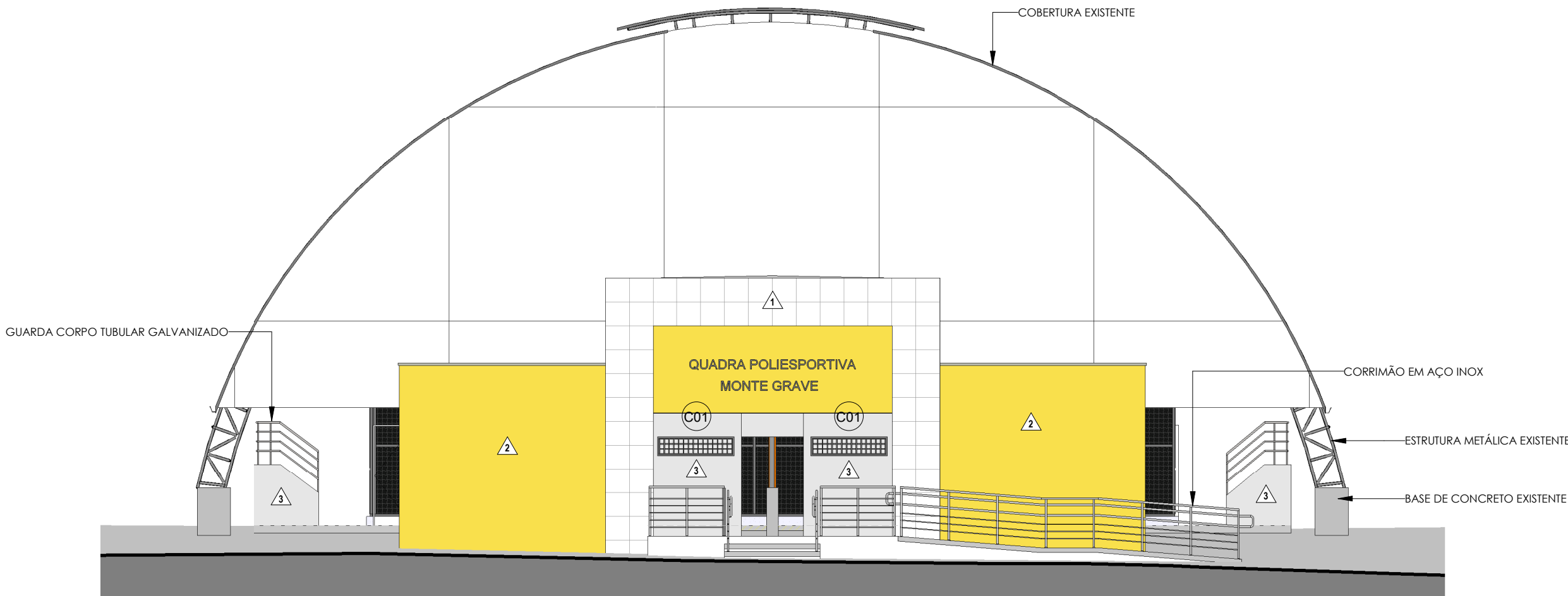
1 FACHADA FRONTAL 1 : 100
