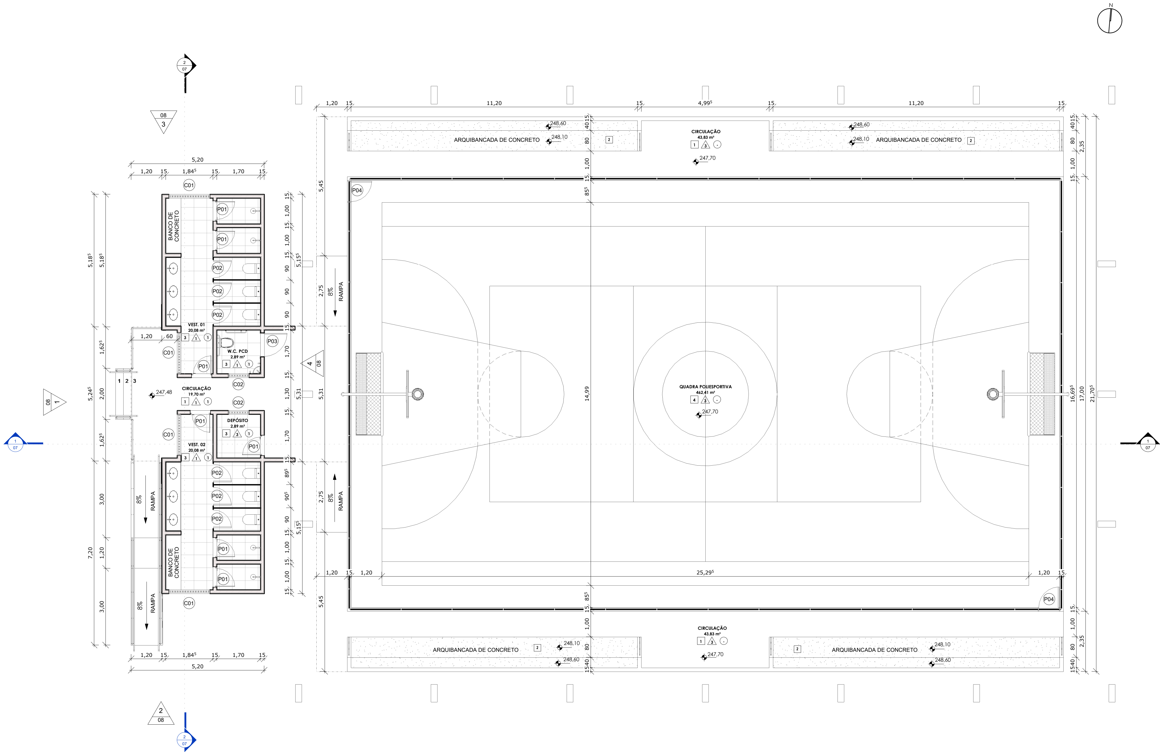
1 | PLANTA BAIXA 1 : 75
