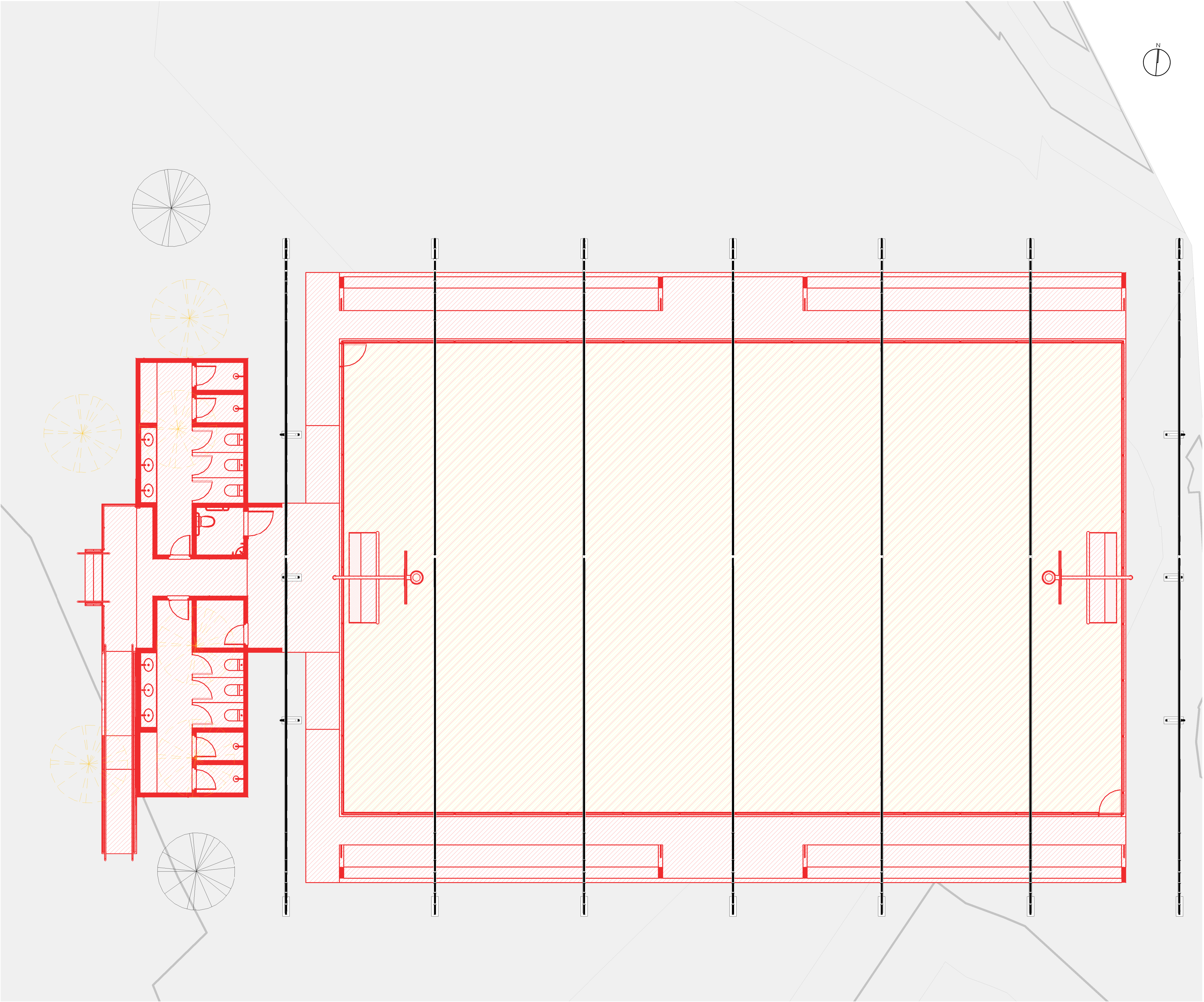
1 | PLANTA BAIXA - CONSTRUIR / DEMOLIR 1 : 75
