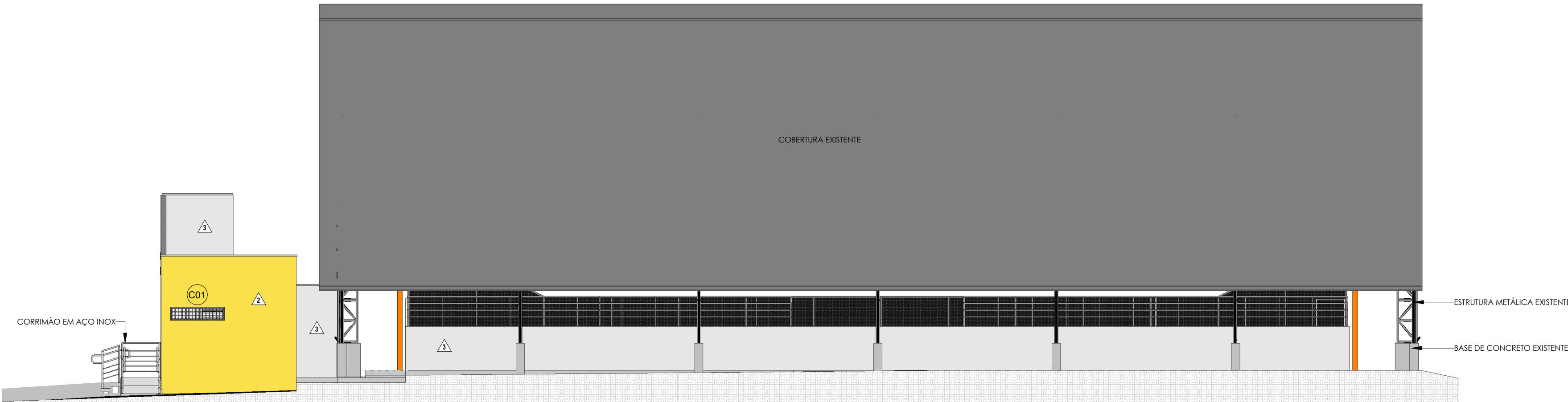
2 FACHADA LATERAL 01 1 : 100
