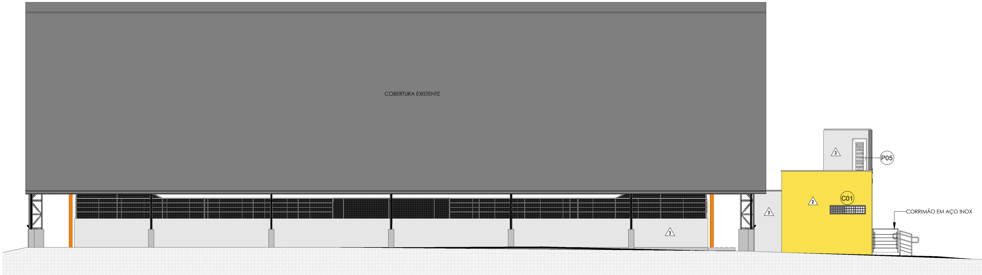
3 FACHADA LATERAL 02 1 : 100
