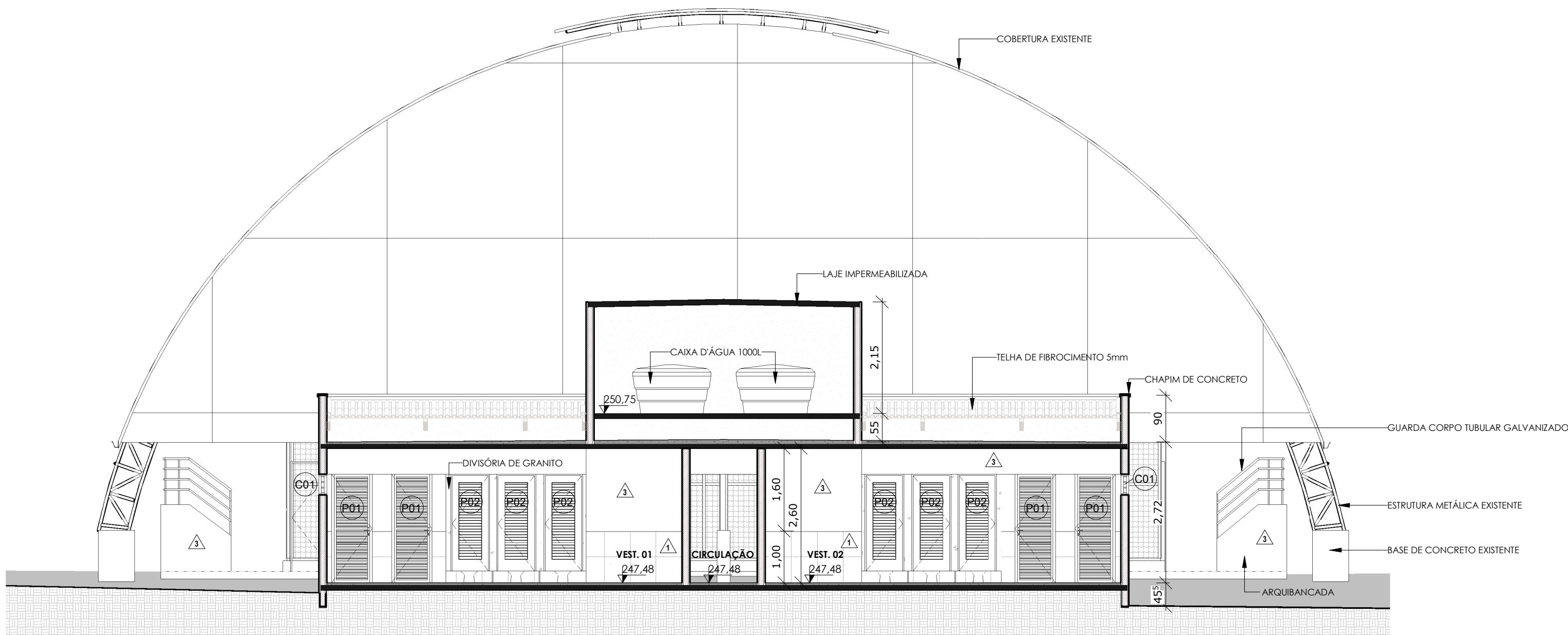
2 | CORTE 02 1 : 75
