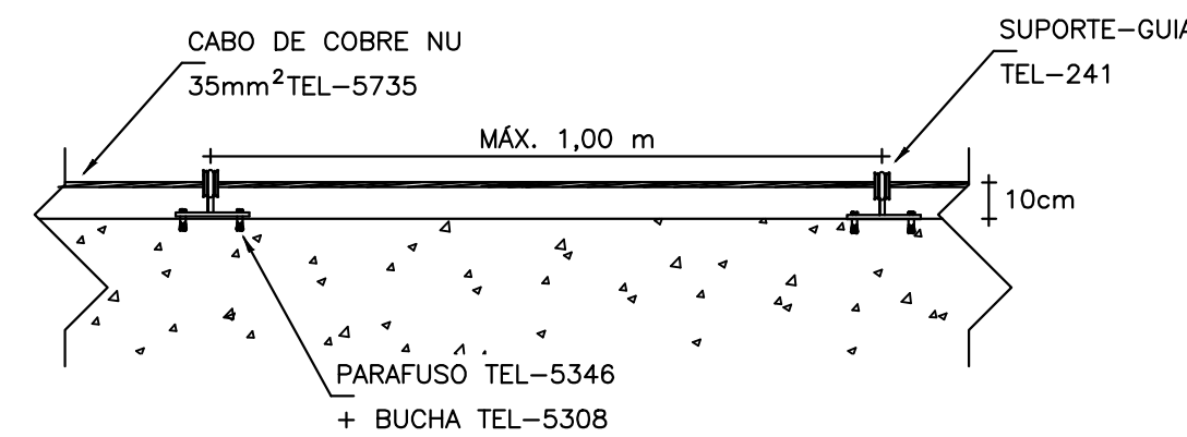
CABO FIXADO ATRAVÉS DE SUPORTE GUIA CURTO DETALHE 12 SEM — ESCALA
