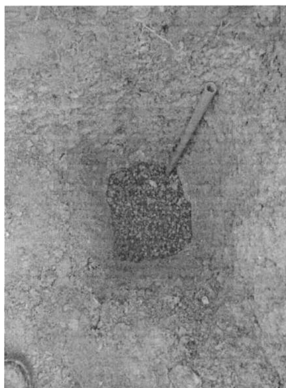
FOTO 3 – VALA PREPARADA PARA O TESTE DE ABSORÇÃO
