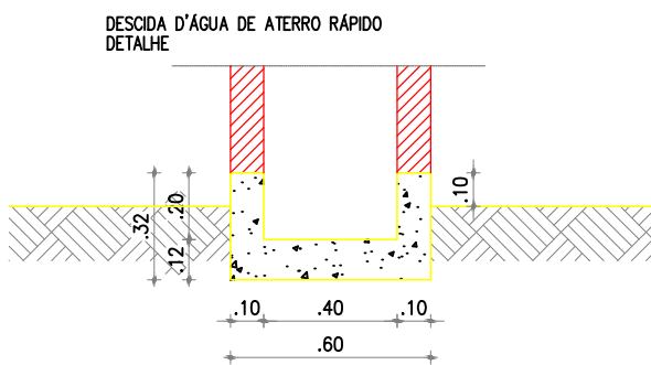
05 CORTE Z-Z DESCIDA D'ÁGUA ESCALA: 1/20
