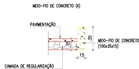
01 DETALHE MEIO-FIO DE CONCRETO ESCALA: 1/20
