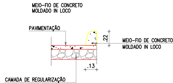
02 DETALHE MEIO-FIO DE CONCRETO ESCALA: 1/20
