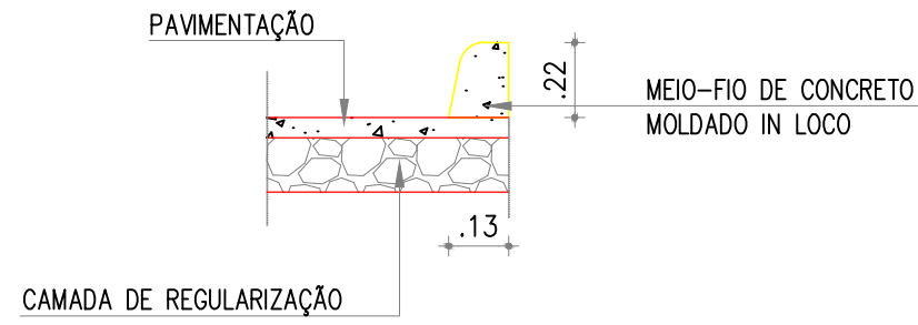
07 DETALHE MEIO-FIO DE CONCRETO ESCALA: 1/20
