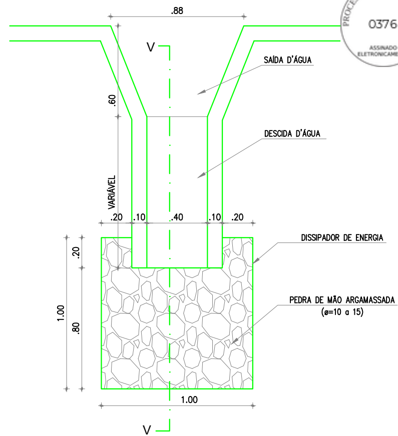
04 PLANTA BAIXA DESCIDA D'ÁGUA E DISSIPADOR DE ENERGIA ESCALA: 1/20
