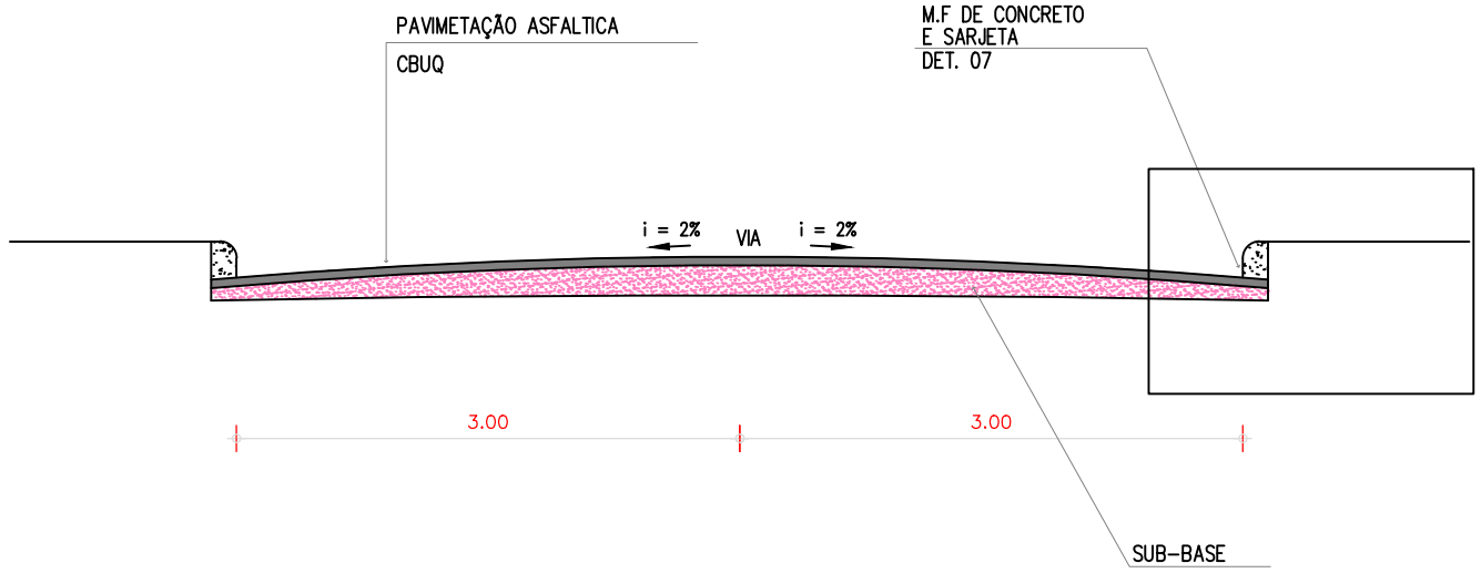
06 SEÇÃO TIPO ESCALA: 1/50
