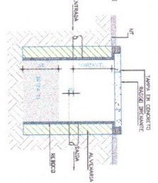
DET 04: CAIXA DE AREIA
