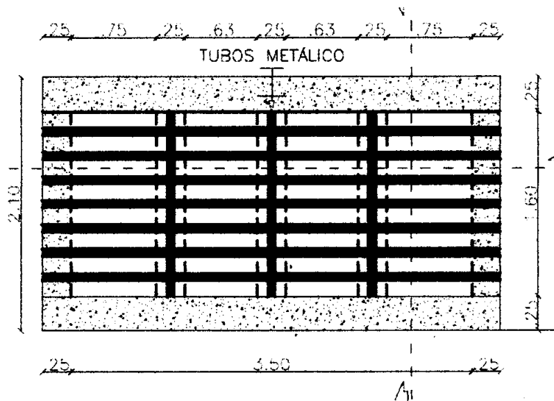
DETALHE LOCALIZAÇÃO DOS TUBOS METÁLICO (GRADE)
