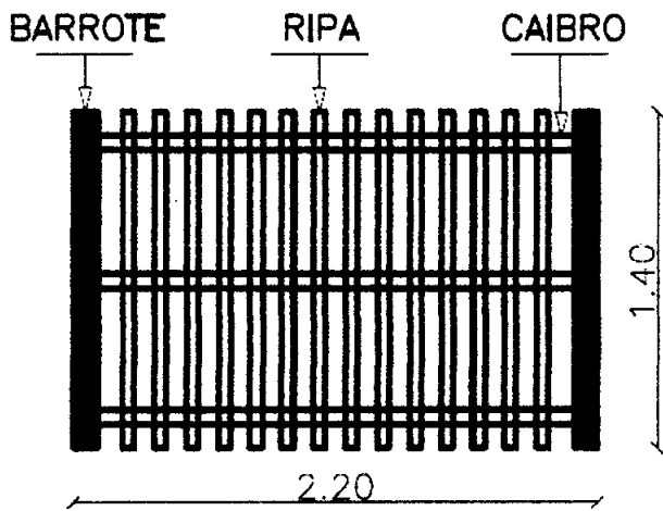
DETALHE DO PORTÃO DE MADEIRA
