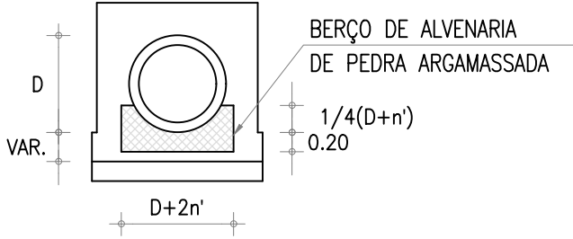
CORTE BB
