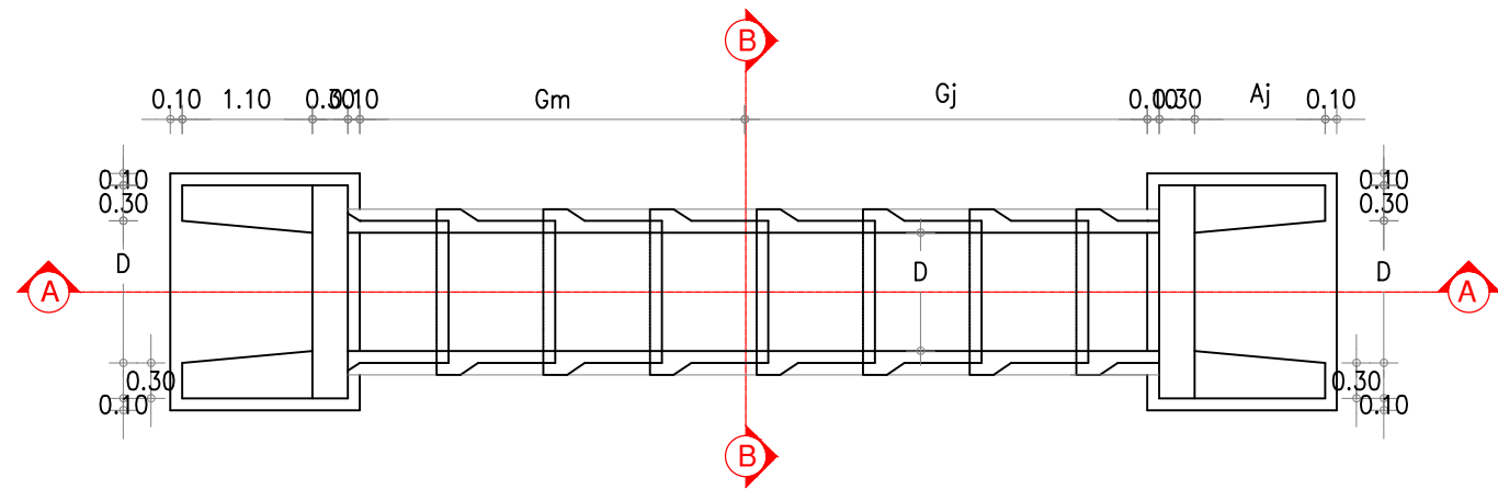
PLANTA BAIXA
