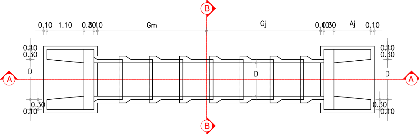
PLANTA BAIXA
