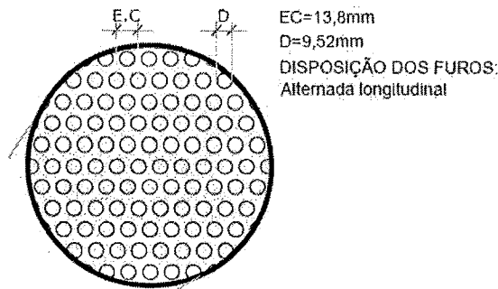
Figura 5 – imagem furos chapa metálica
