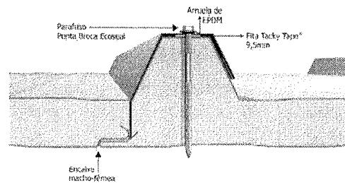
Figura 6 – imagem telha termoacústica
