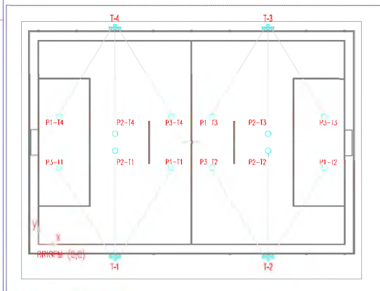
LAYOUT PLANO - POSICIONAMENTO DOS PROJETORES escala: 1/75
