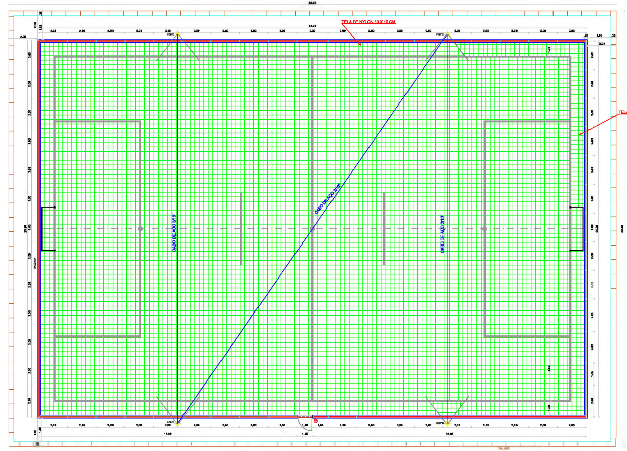
06 PLANTA BAIXA COM TELA DE NYLON
