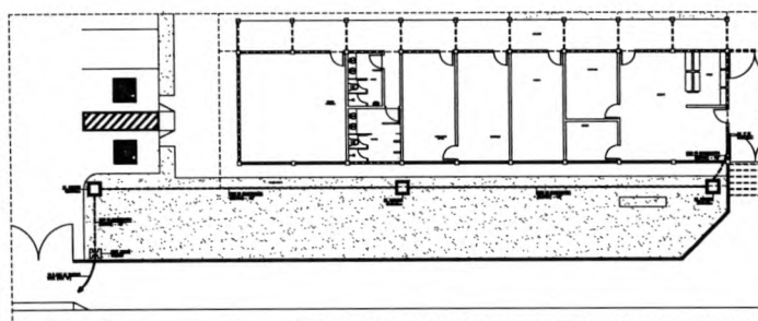
PLANTA BAIXA - LIGAÇÃO escala: 1/100
