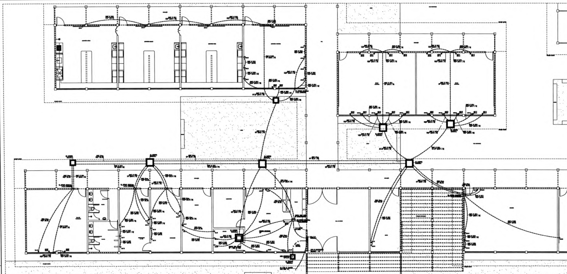
PLANTA BAIXA - TELEFONIA/LÓGICA escala: 1/50
