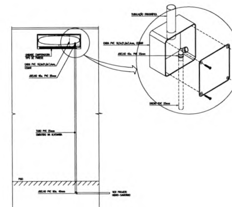
DEALHE DE DRENAGEM SPLIT DE PAREDE
