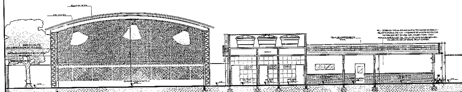
CORTE CC 1:75
