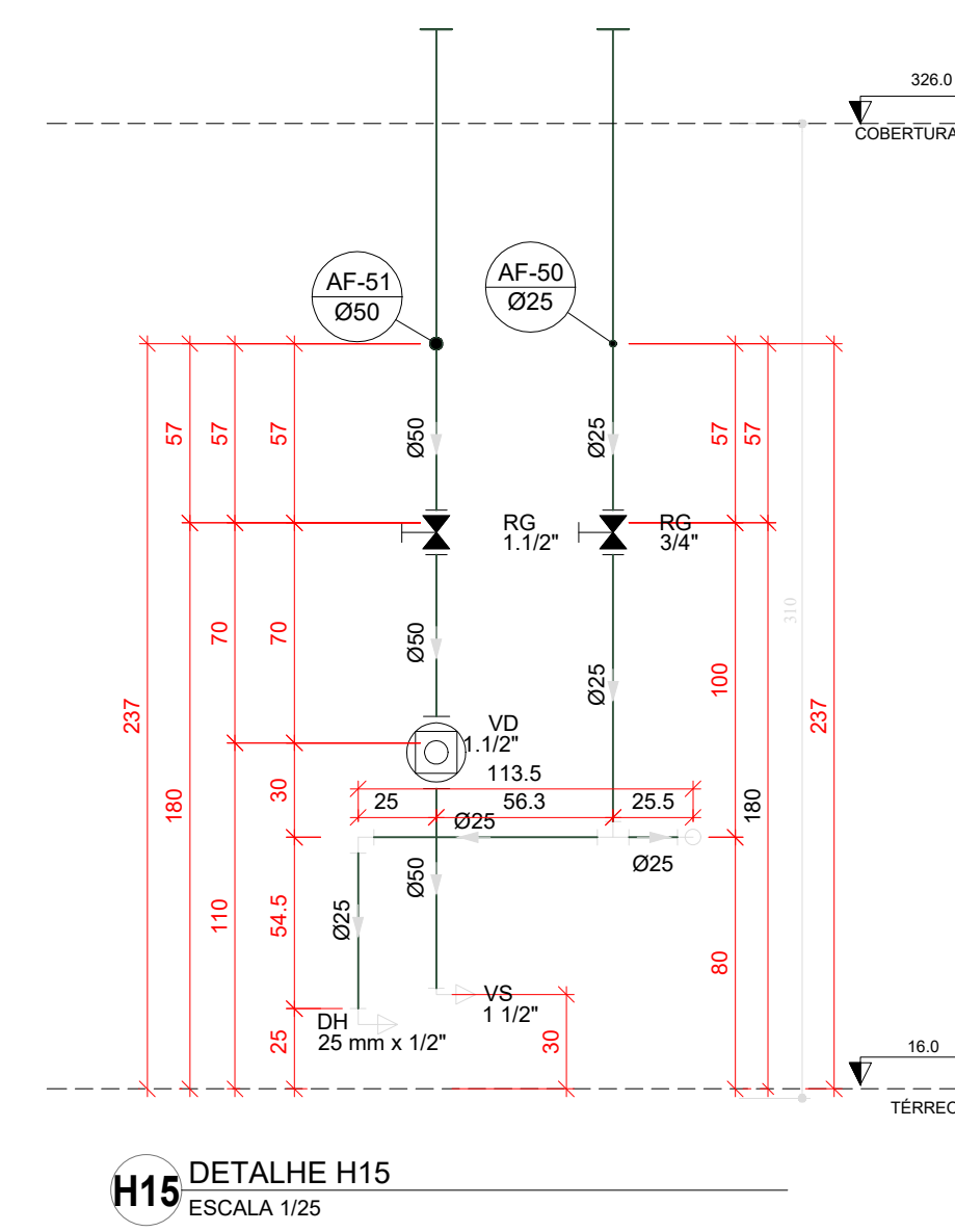
H15 DETALHE H15 ESCALA 1/25
