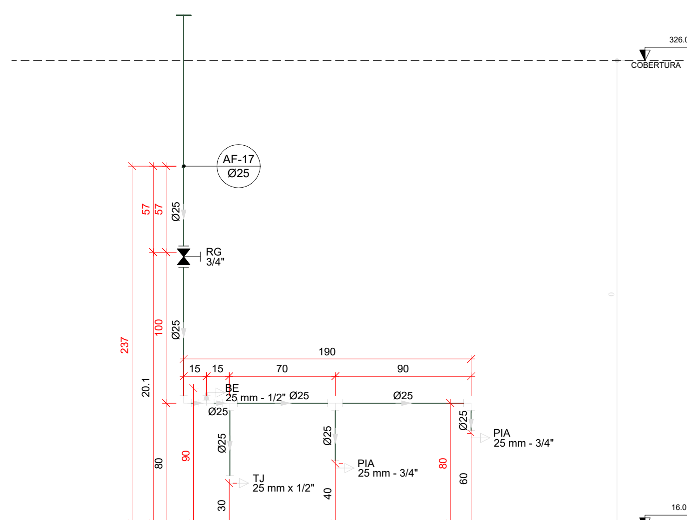
H09 DETALHE H09 ESCALA 1/25
