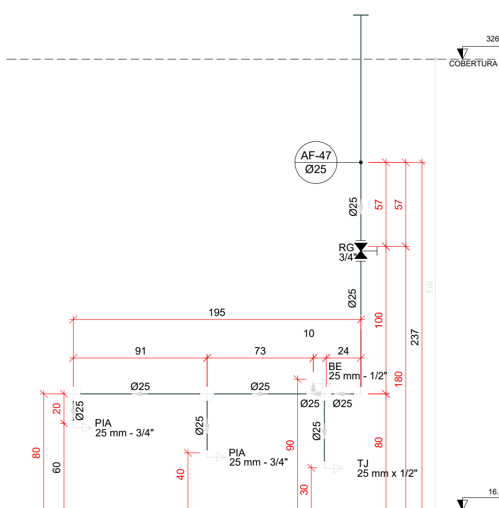
H11 DETALHE H11 ESCALA 1/25
