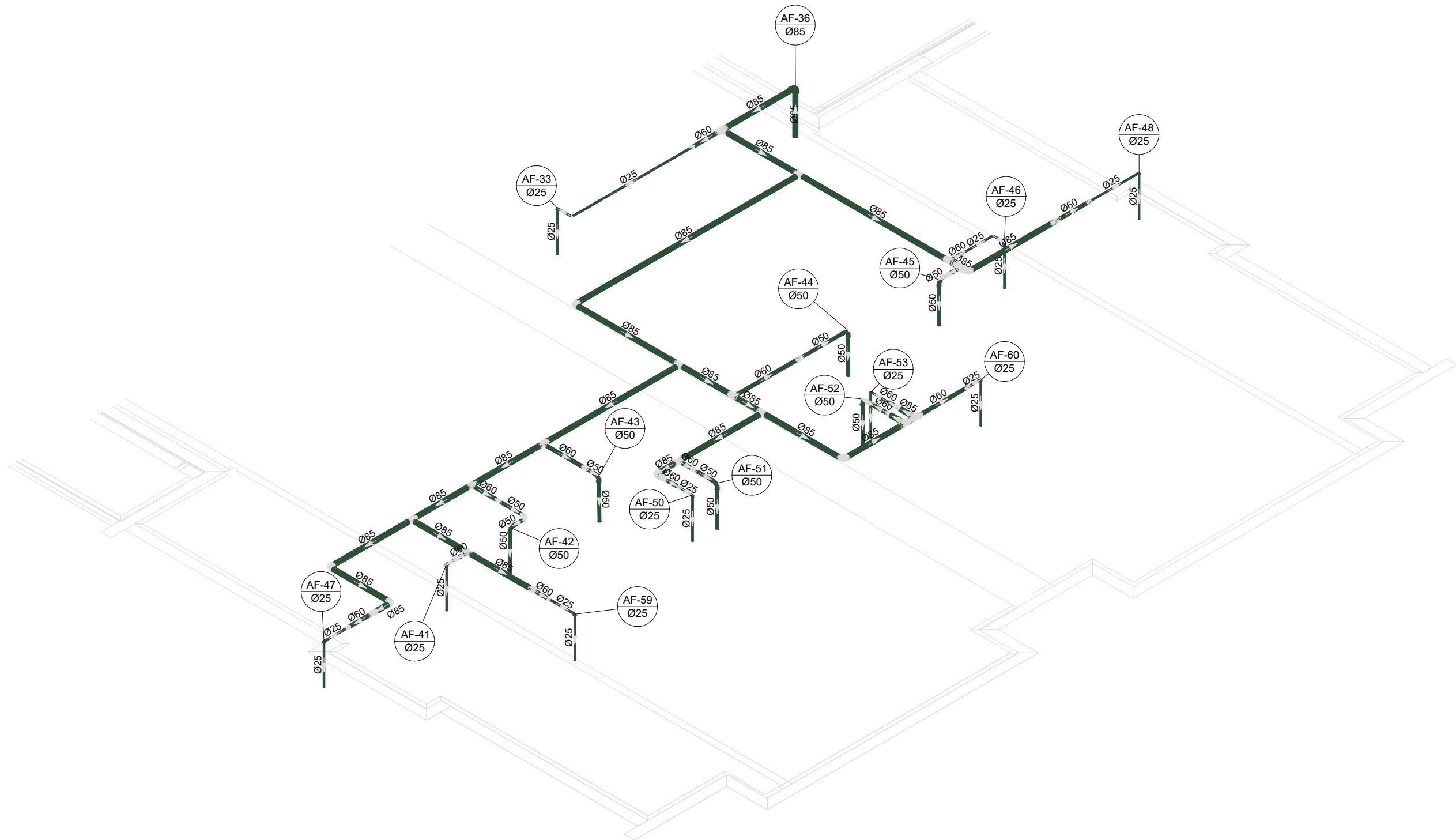
D40 DETALHE ISO 40 ESCALA 1/75
