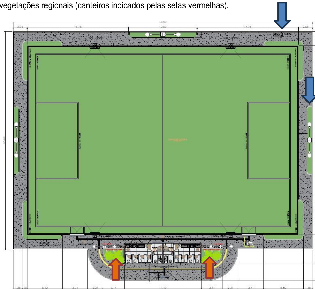
Figura 05: Planta baixa da Areninha. Fonte: Acervo próprio.
