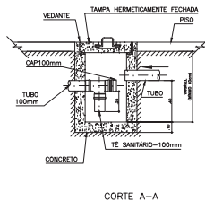
CAIXA DE GORDURA/SABÃO ESCALA: 1:1
