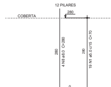
P3=P4=P5=P6=P10=P11=P12=P13=P17=P18=P19=P20 12 BASES PLANTA - S4
