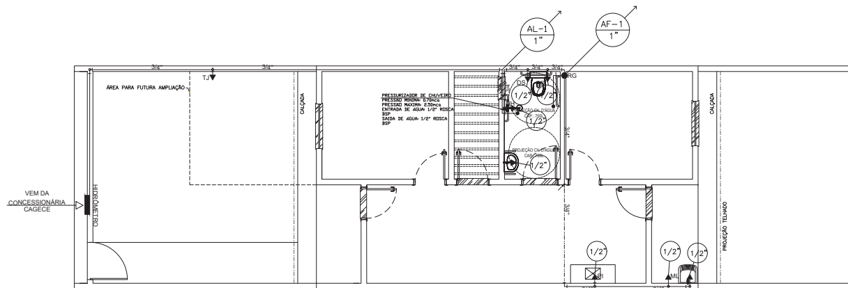
01 PROJETO HIDRÁULICO ESCALA: 1/50
