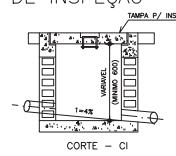
DETALHE CAIXA DE INSPEÇÃO
