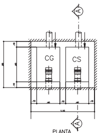
CAIXA DE GORDURA/SABÃO ESCALA: 1:1
