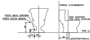
–DETALHE BACIA SANITARIA COM CAIXA ACOPLADA – DUCHA MANUAL
