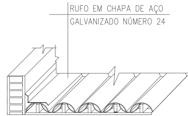
05 DETALHE RUFO 050 ESCALA
