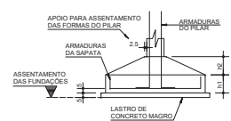
ARRANQUE DOS PILARES EM SAPATAS
