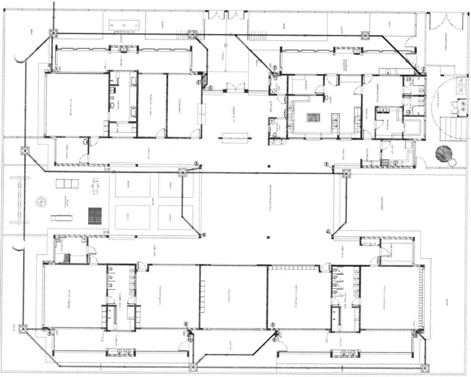
1 PLANTA BAIXA ESCALA 1/76
