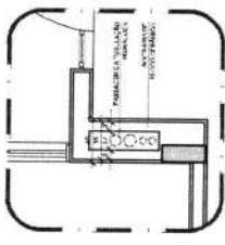
2 DETALHE - SHAFT HIDRAULICA ESCALA 1/25
