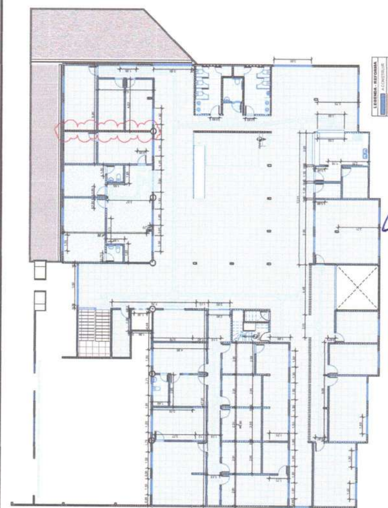
2 REFORMA PAV. 1 - PL. B. DEN/CONSTR. FORMA 1:100
