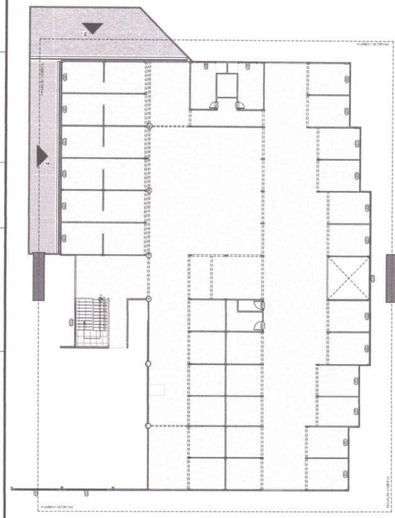
1 PL. B. PAV. 1 - EXISTENTE FORMA 1:100
