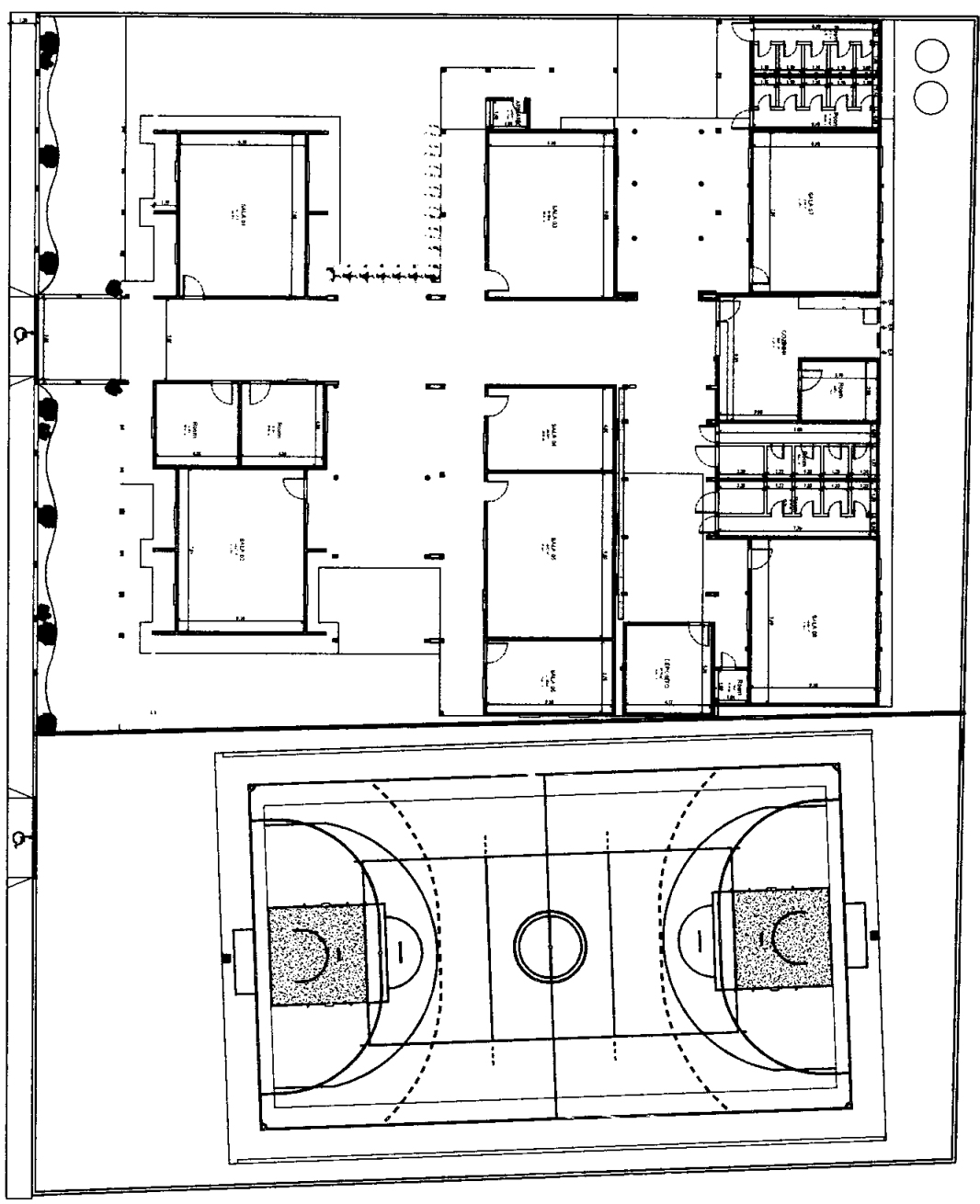
1 PLANTA BANHA - COTAS Escala: 1:100
