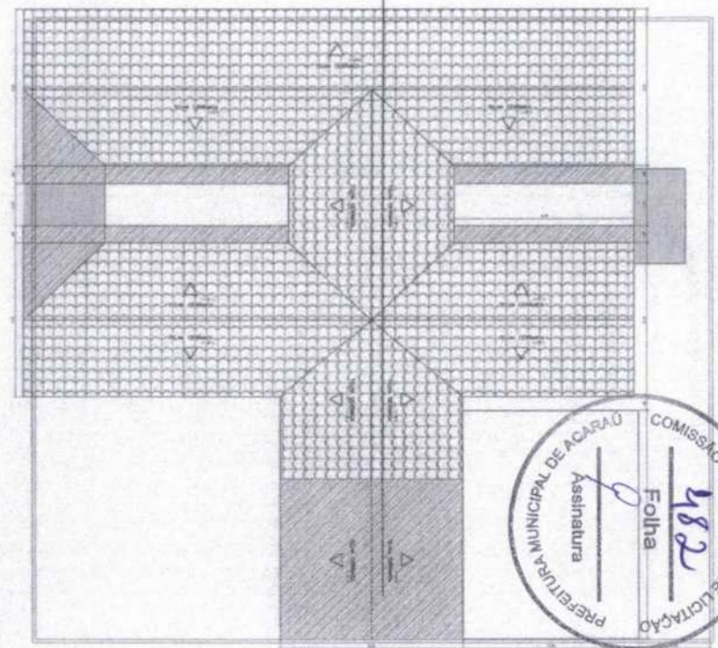
02 DEMOLIÇÃO E CONSTRUÇÃO ESCALA 1/100
